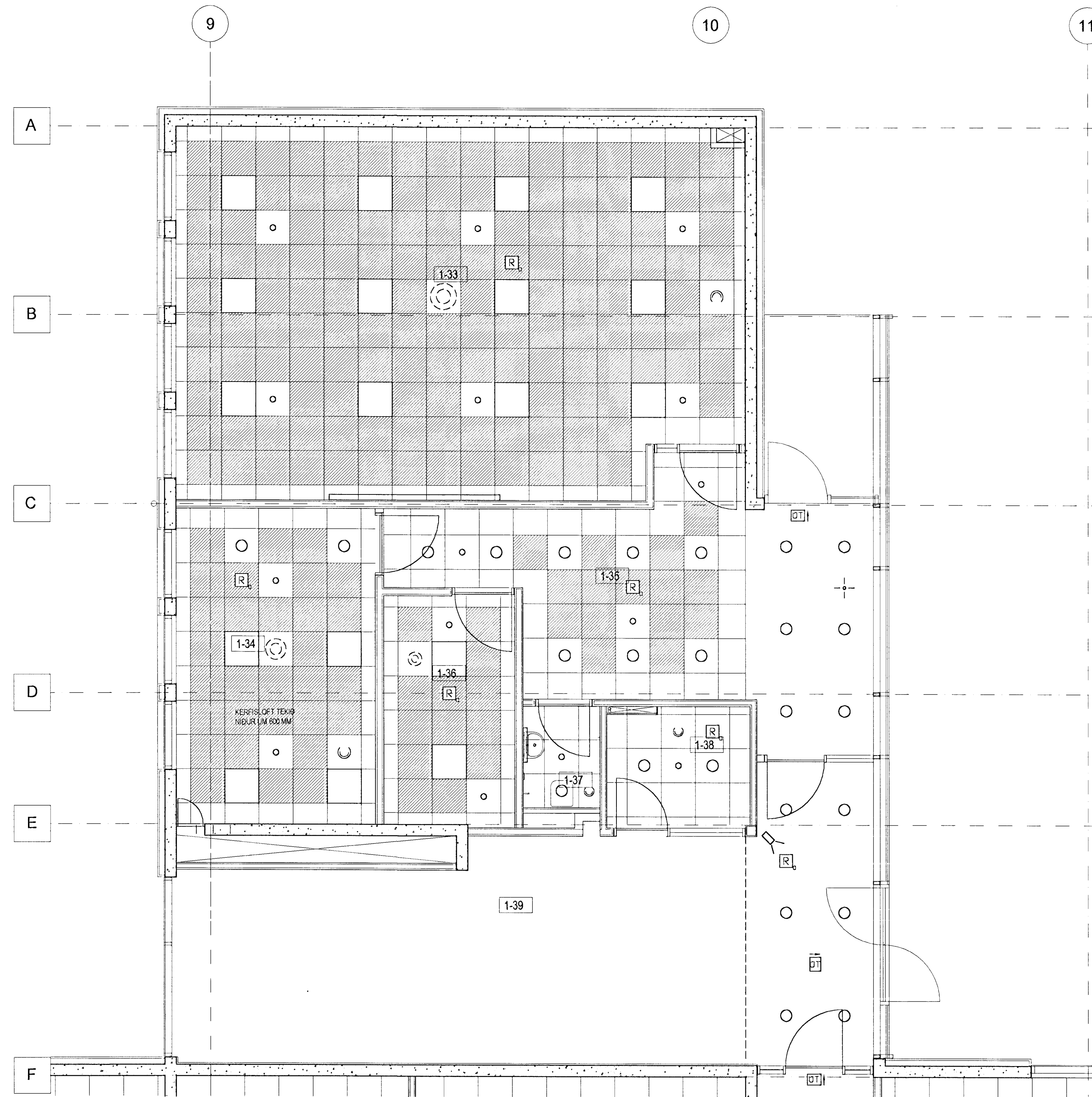
GRUNNMYND JARÐHÆÐAR 1:50, ÞVERÁLMA
