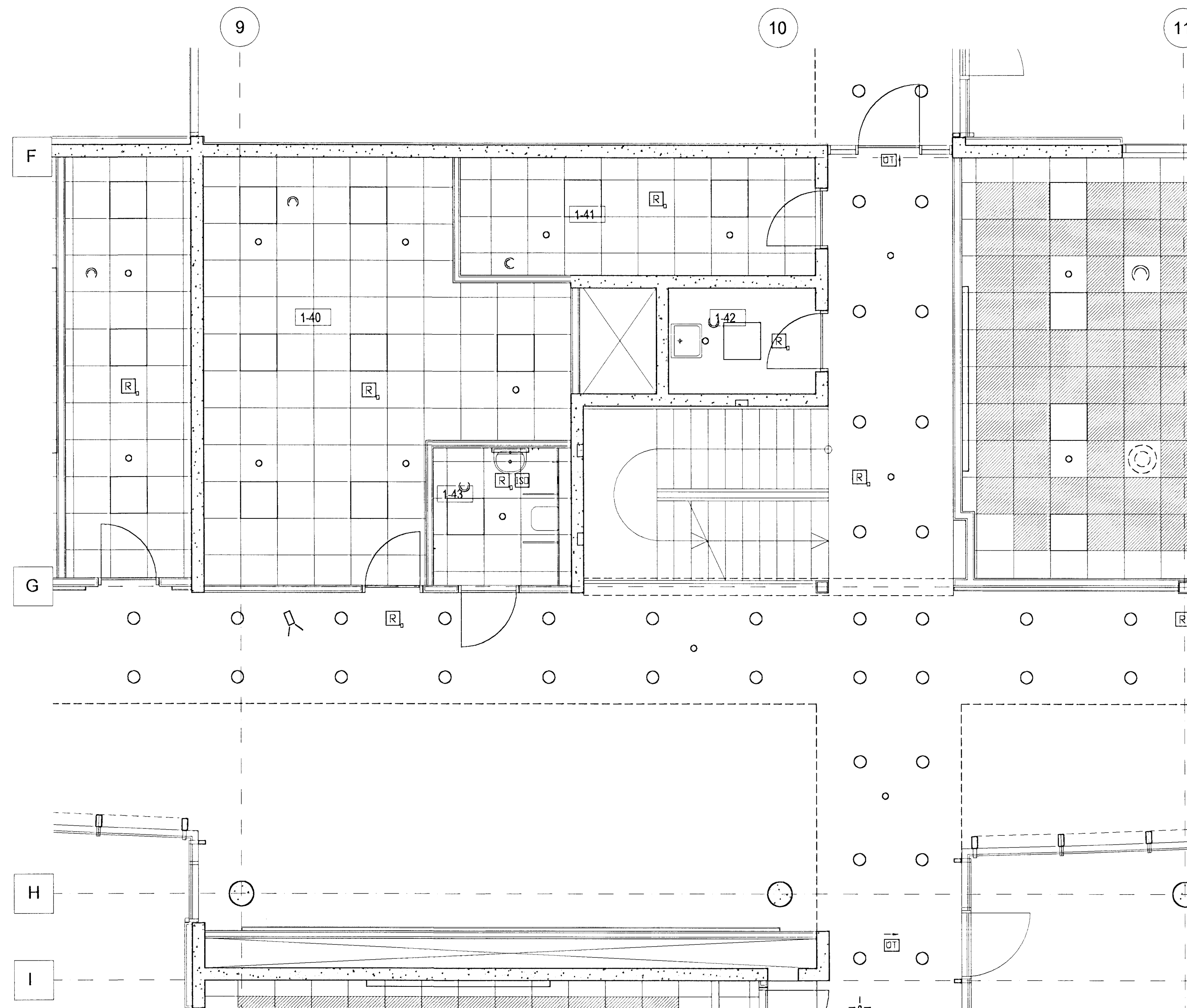
GRUNNMYND 1. HÆÐAR 1:50, AÐALÁLMA
