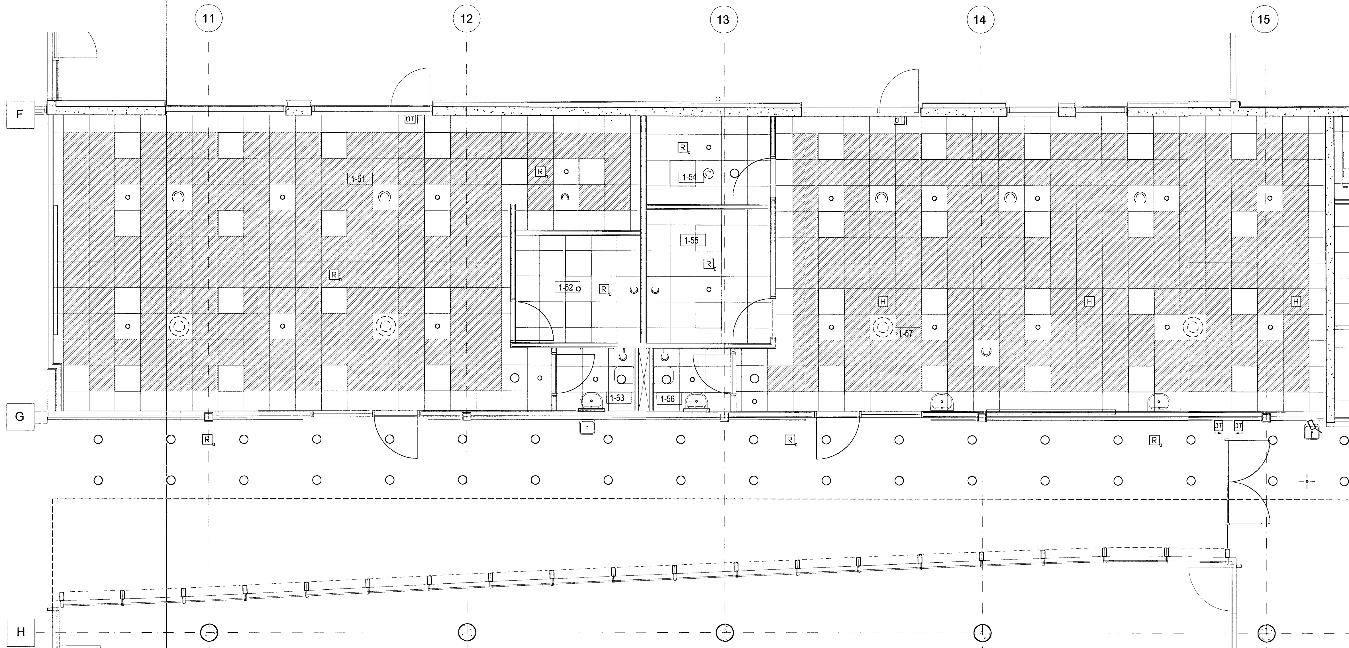
GRUNNMYND 1. HÆÐAR 1:50, ADALÁLMA
