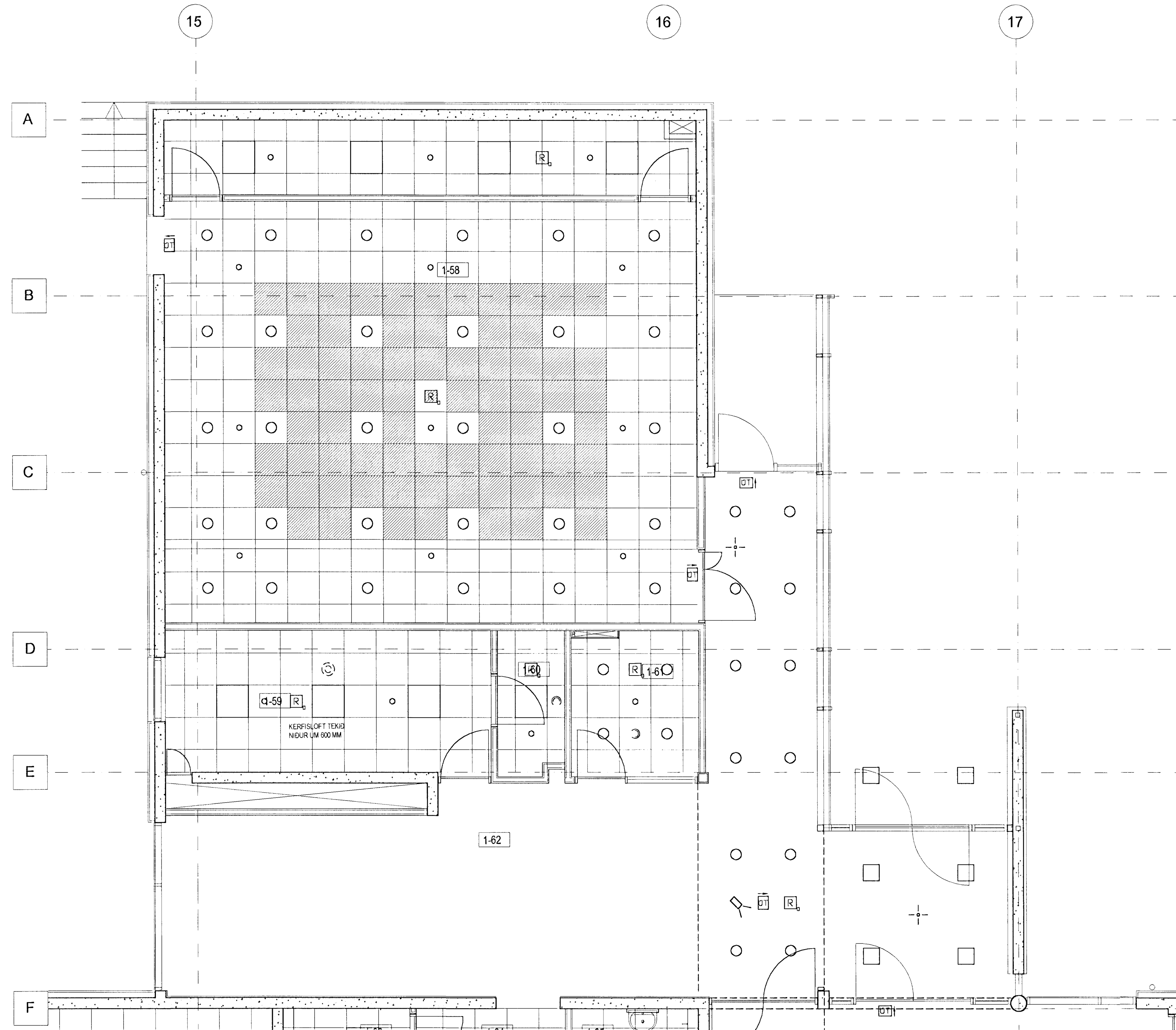
GRUNNMYND 1. HÆÐAR 1:50, ÞVERÁLMA
