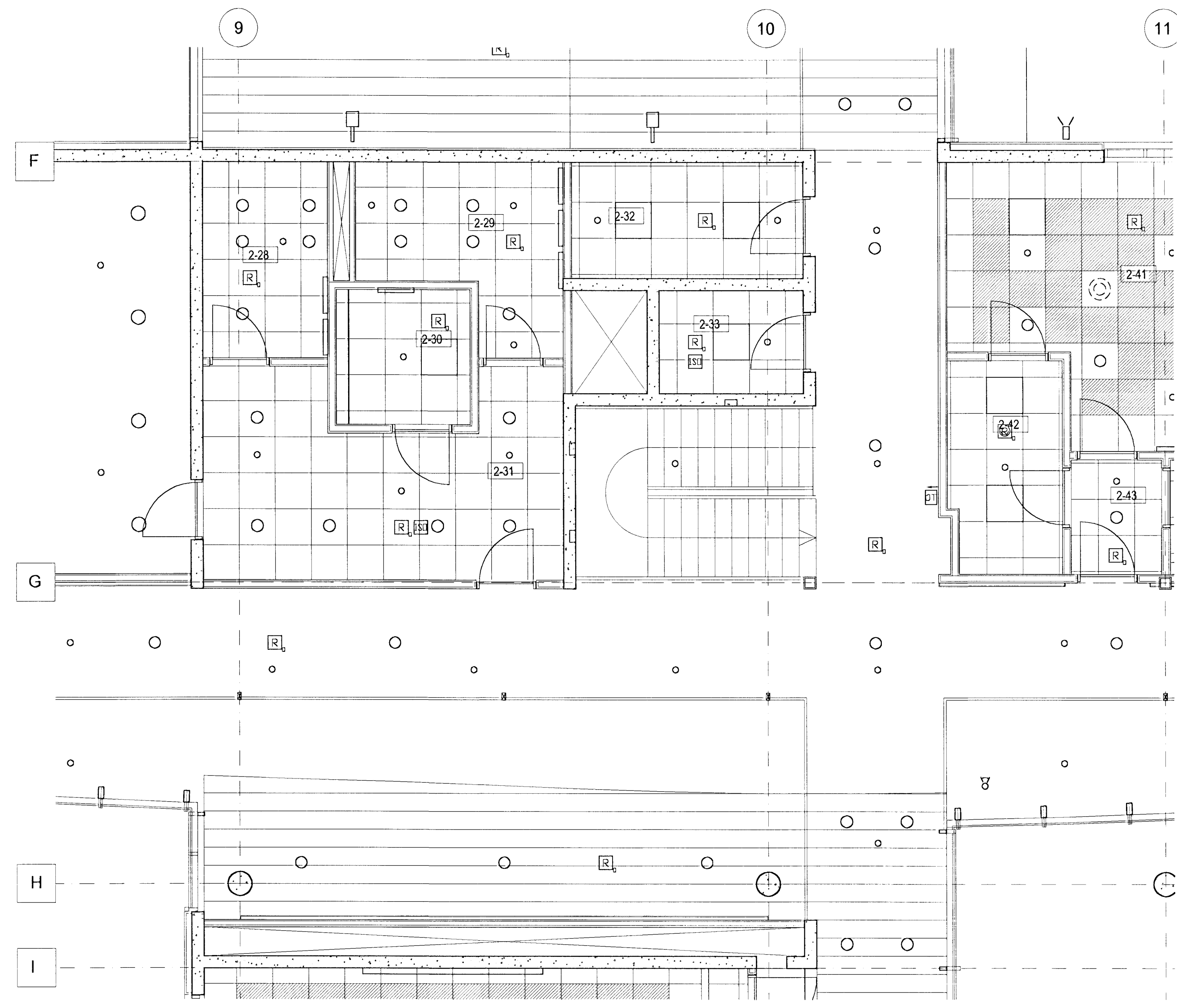
GRUNNMYND 2. HÆÐAR 1:50, AÐALÁLMA
