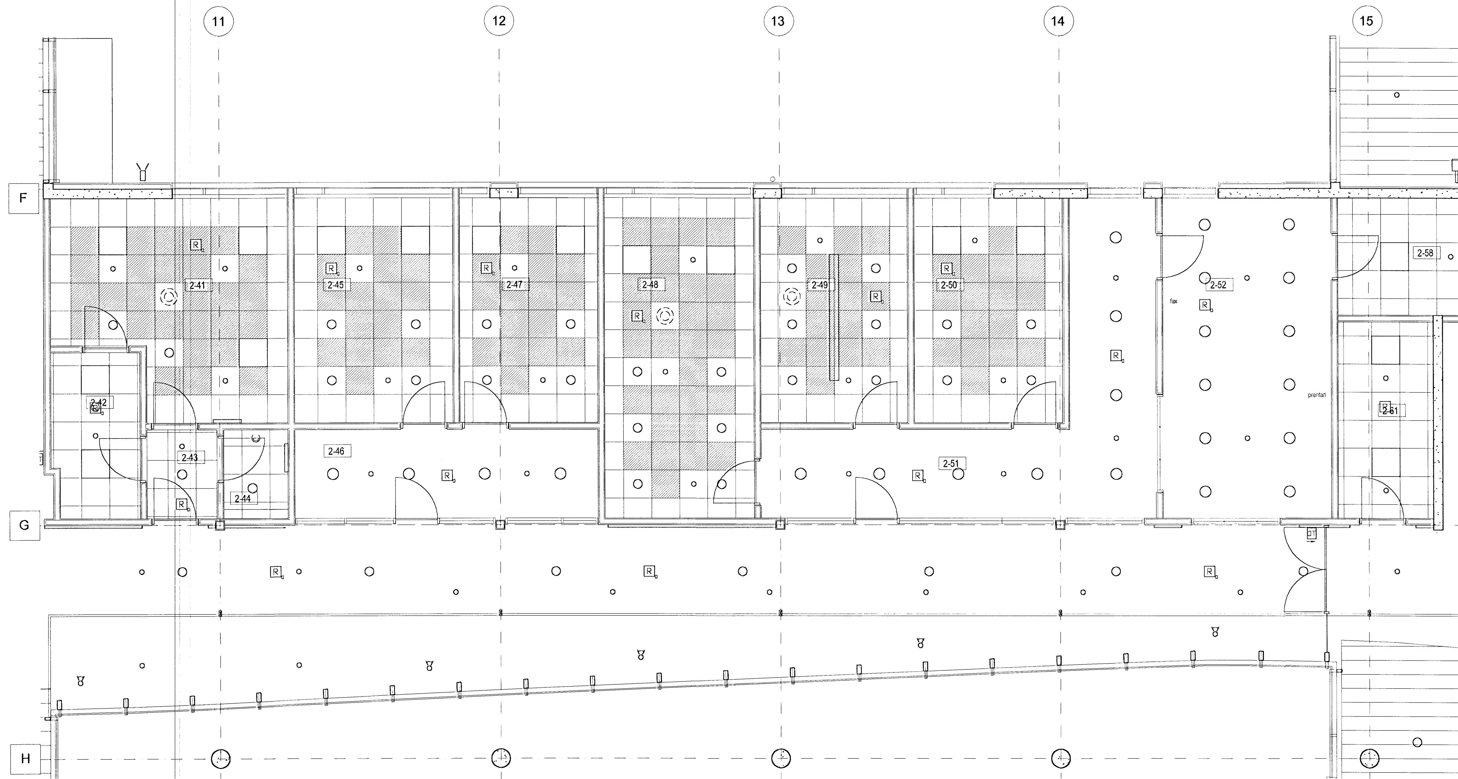
GRUNNMYND 2. HÆÐAR 1:50, ADALÁLMA
