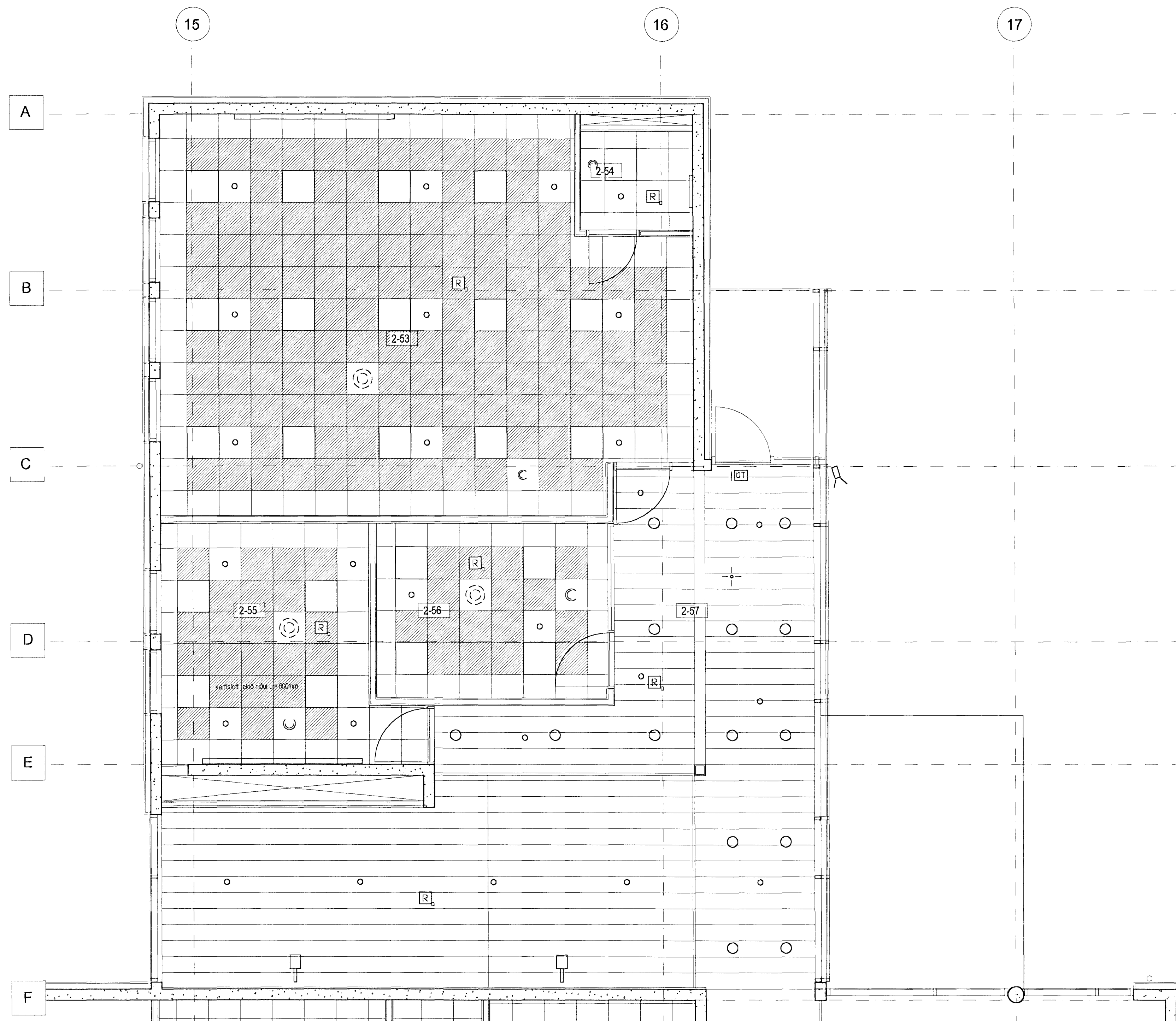
GRUNNMYND 2. HÆÐAR 1:50, ÞVERÁLMA
