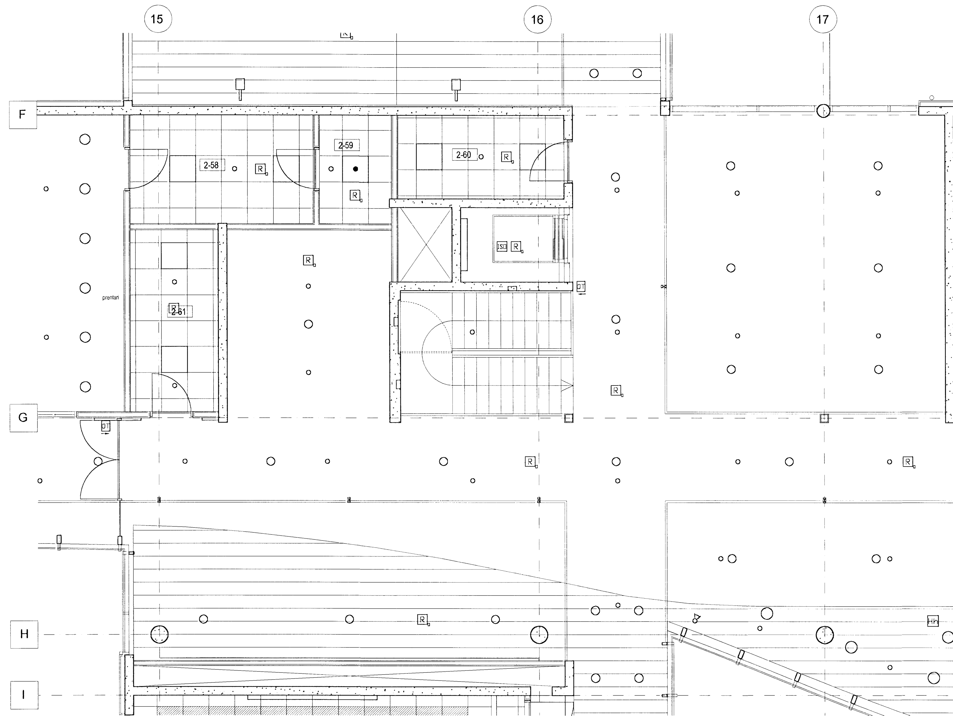
GRUNNMYND 2. HÆÐAR 1:50, AÐALÁLMA
