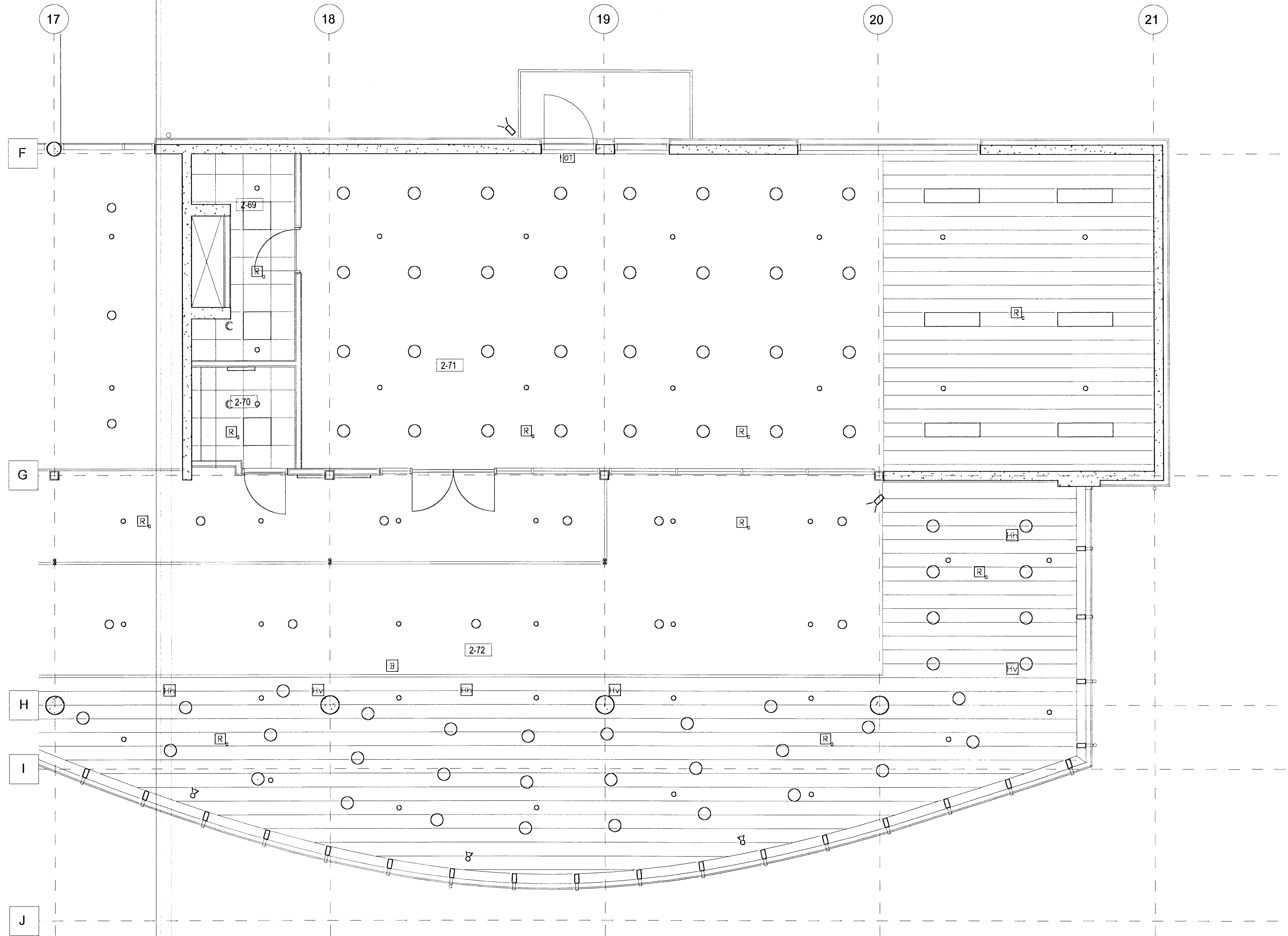
GRUNNMYND 2. HÆÐAR 1:50, ADALÁLMA
