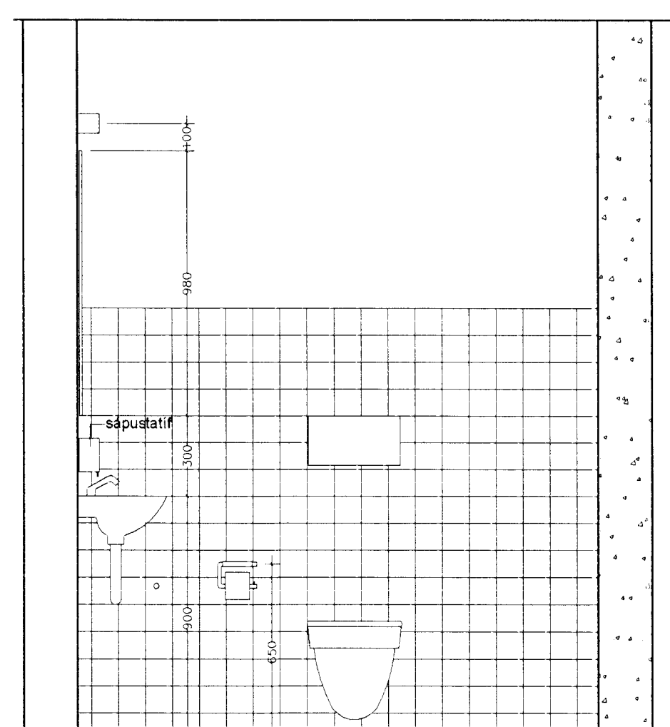
ÁSÝND B.B, RÝMI 1-65
