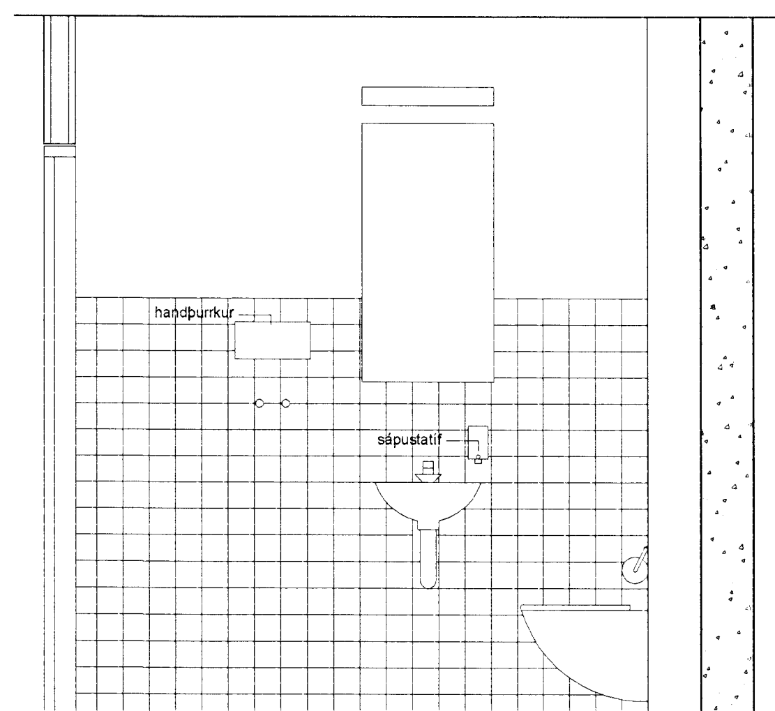
ÁSÝND A.A, RÝMI 1-65
