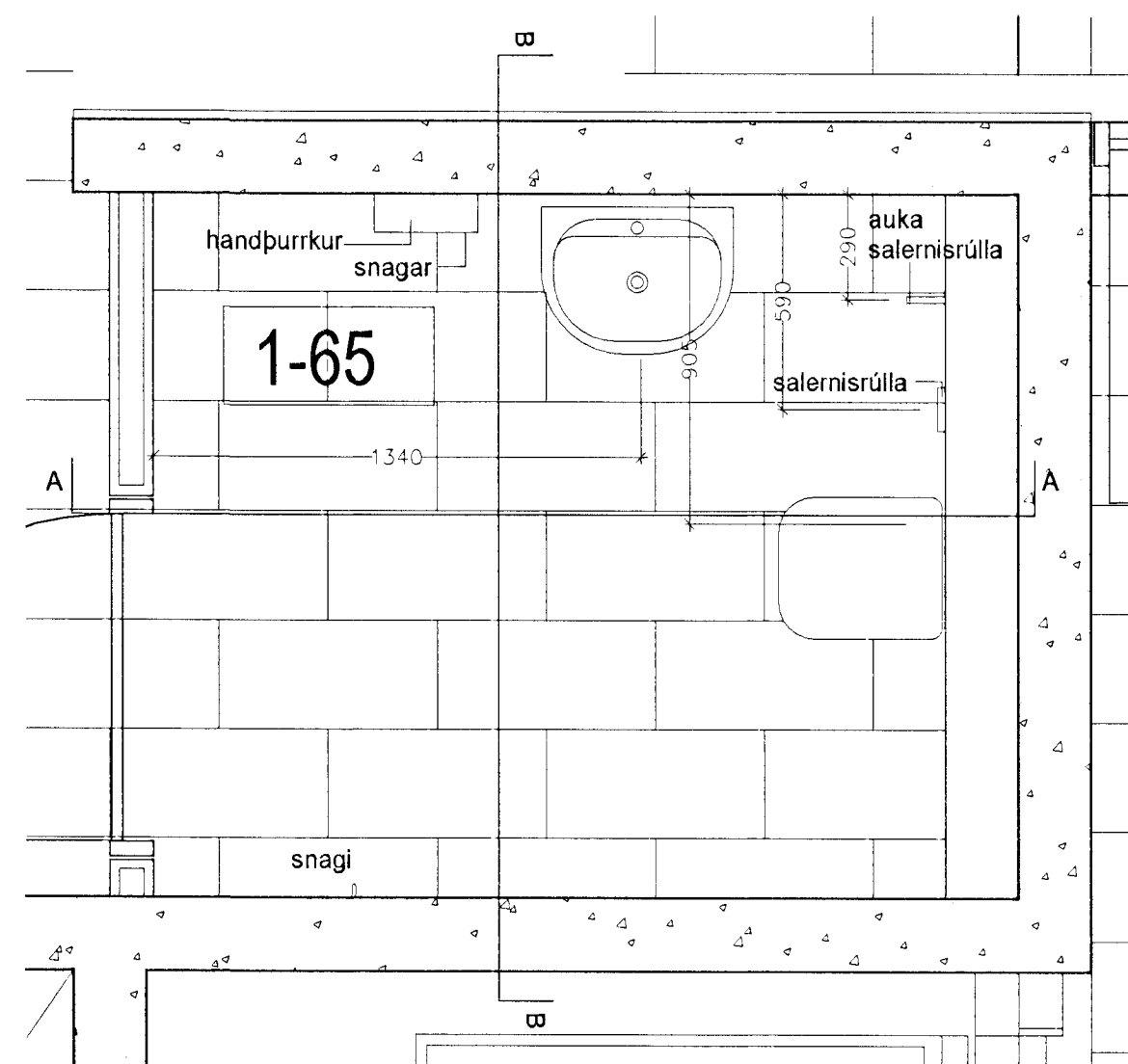
GRUNNMYND RÝMI 1-65 SNYRTING FATLAÐRA
