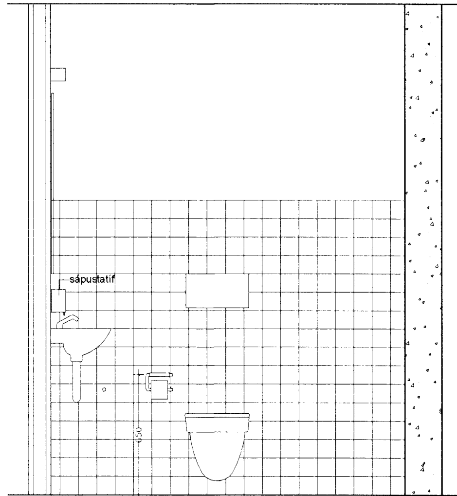
ÁSÝND B.B, RÝMI 1-63
