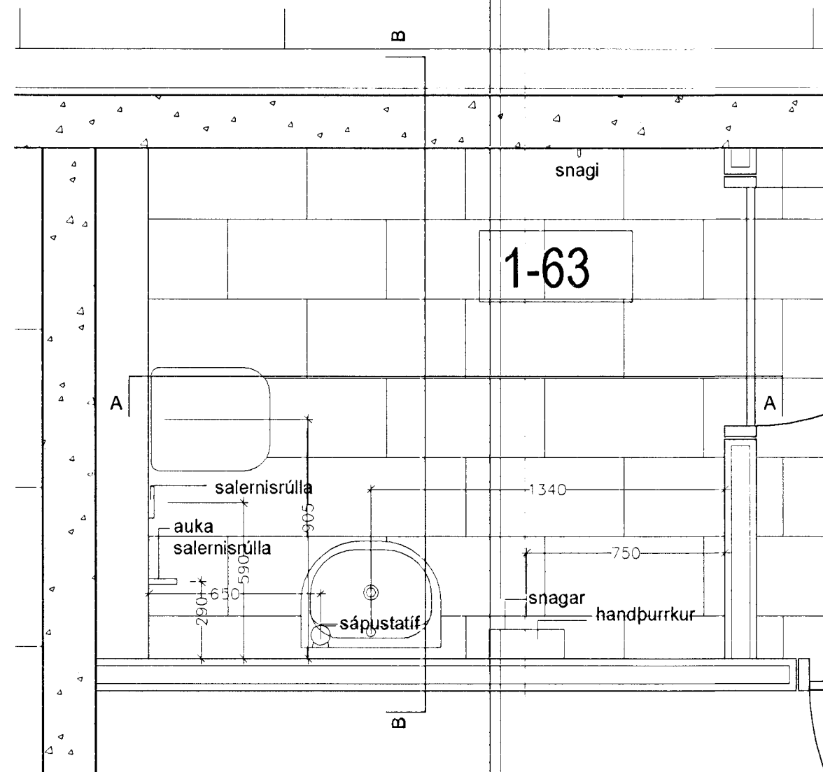
GRUNNMYND RÝMI 1-63 SNYRTING FATLAÐRA
