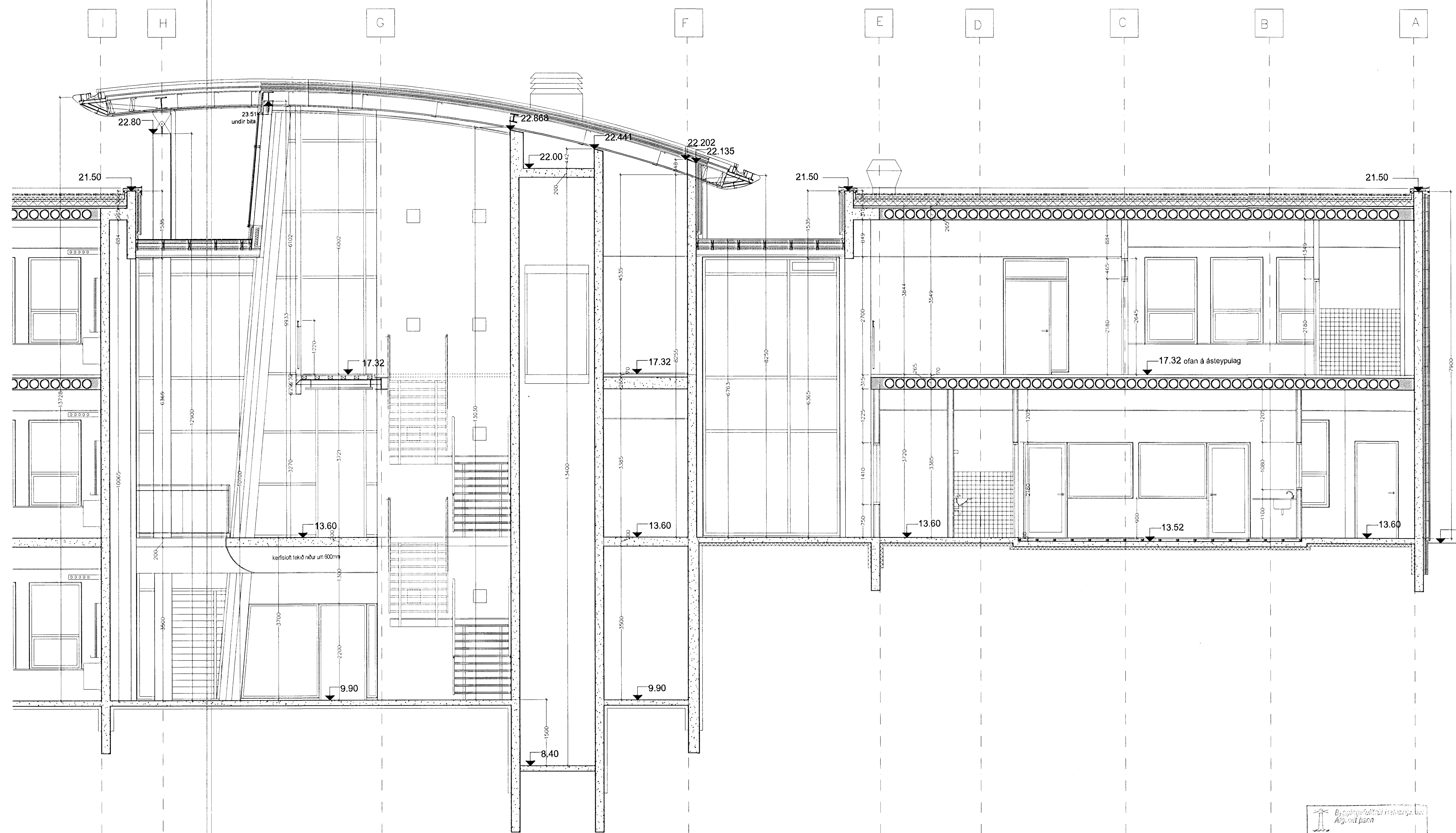
ÞVERSNIÐ A:A
