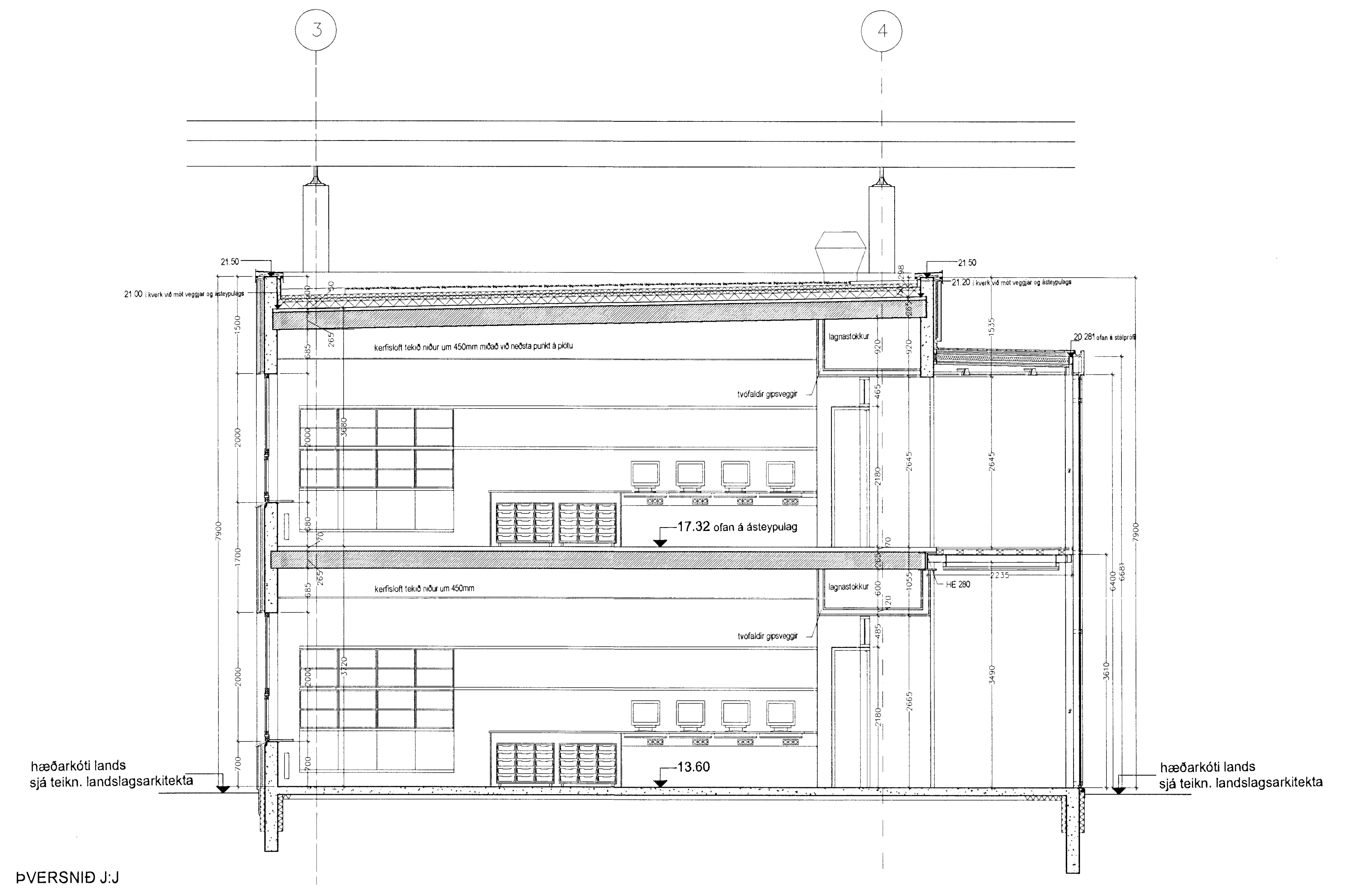
ÞVERSNIÐ J:J
