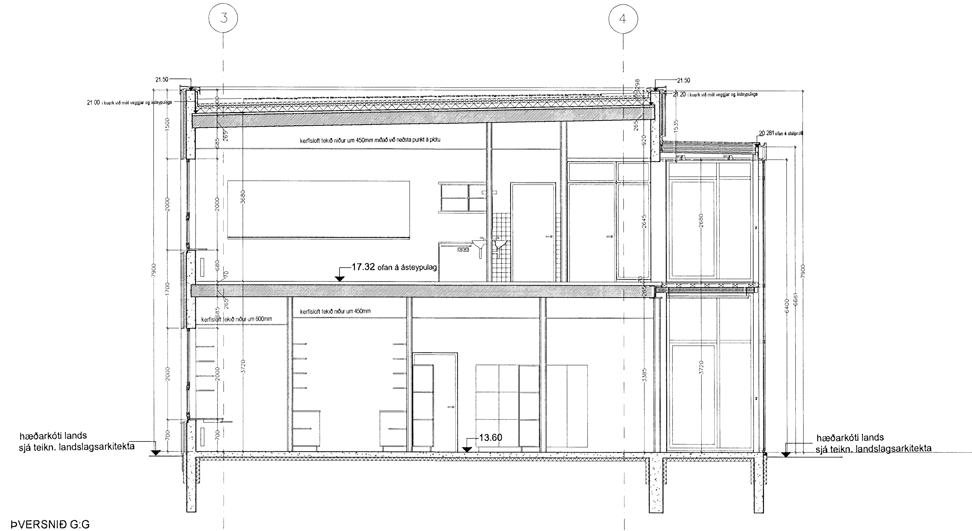
ÞVERSNIÐ G:G
