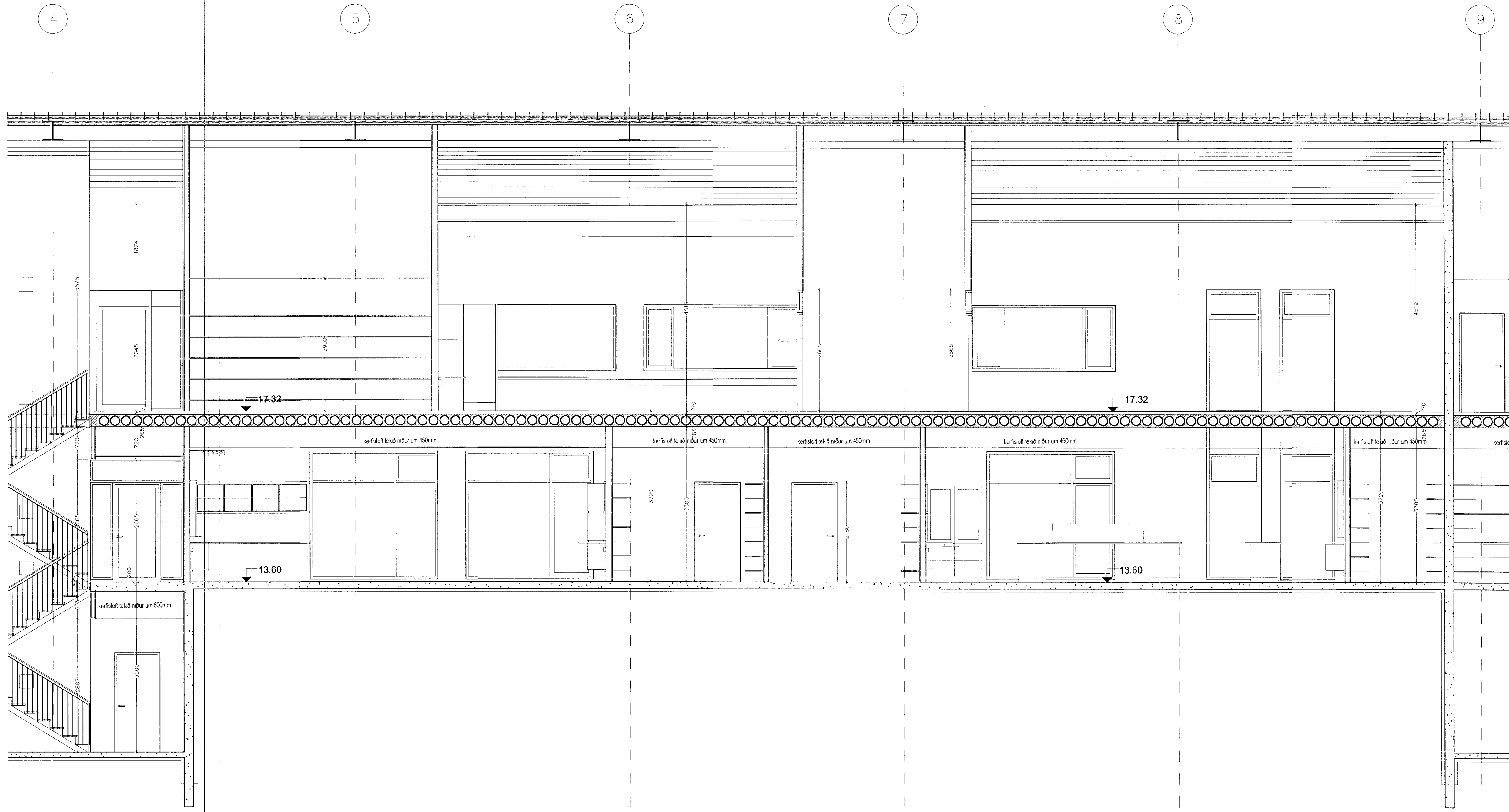
LANGSNIÐ H:H
