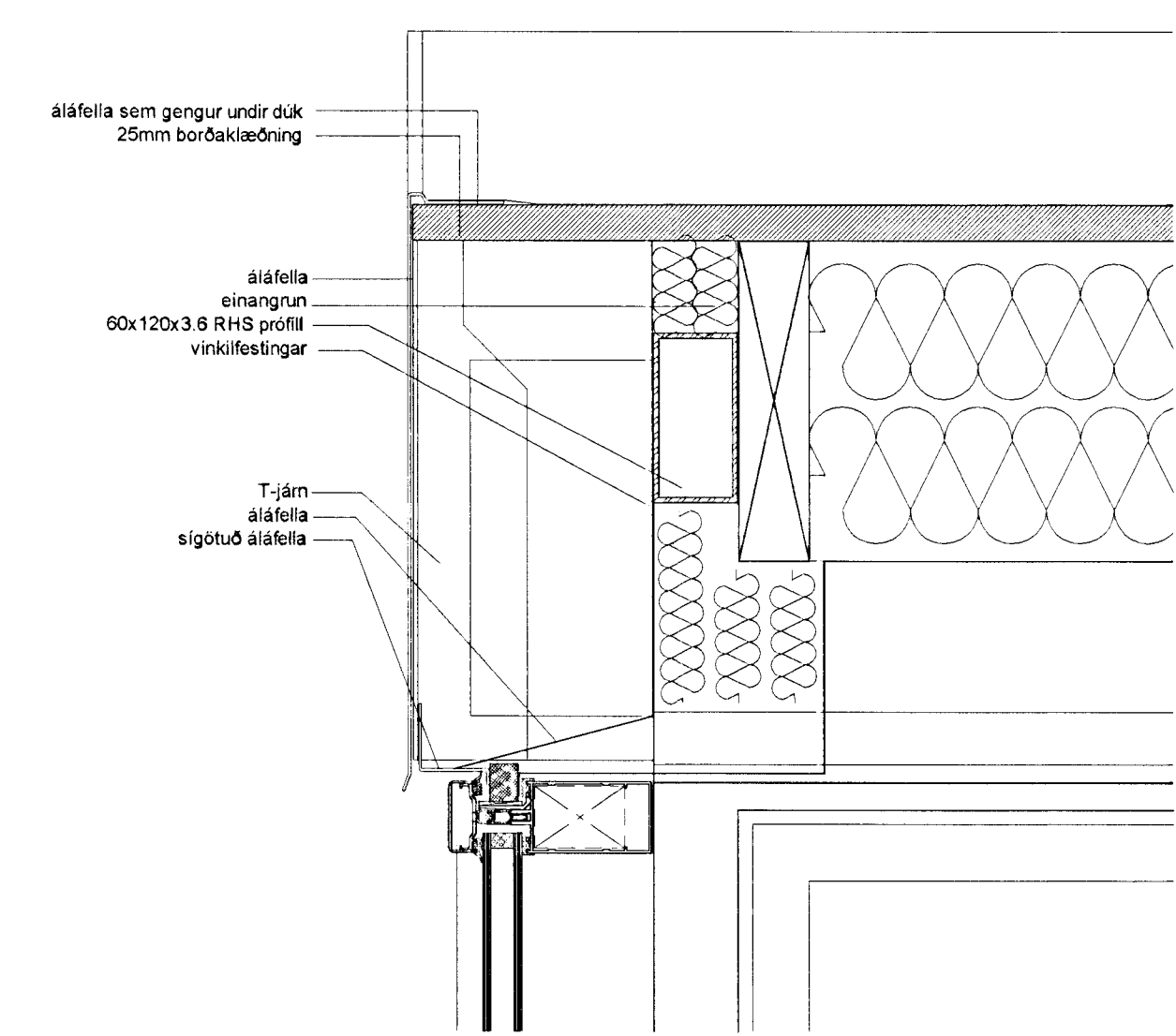
Langsnið í gleranga við þverálmur, frágangur við gaffa
