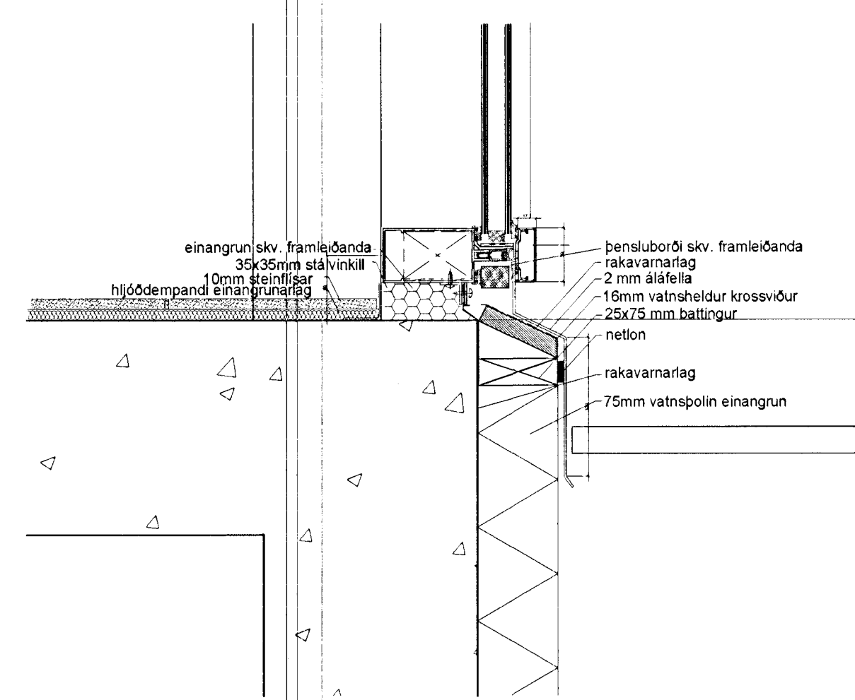
Þversnið í gleranga við þverálmur, frágangur við gólf
