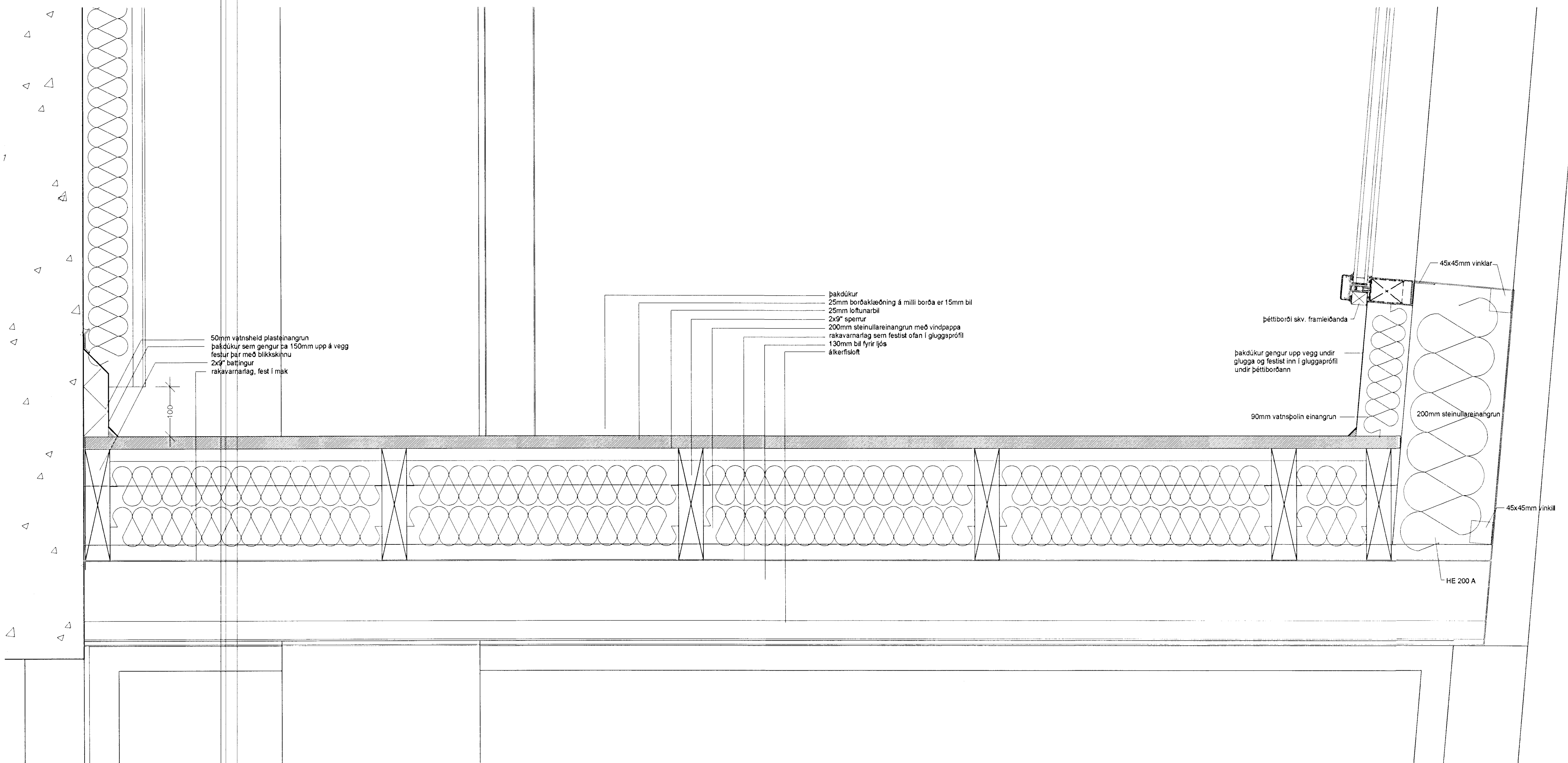
Þversnið í millipak á milli þverálma og bogaveggjar
