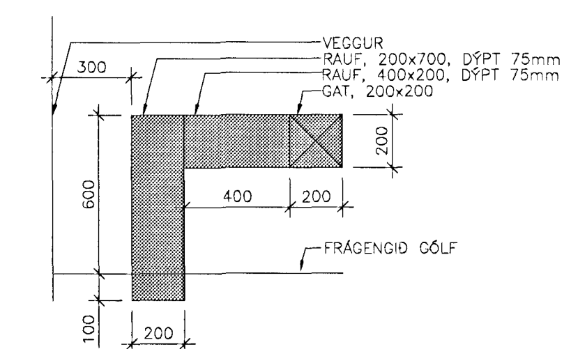
SM1 VEGGRAUF 2, (VR2) 1:20
