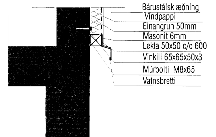
Mkv 1:10 D-D
