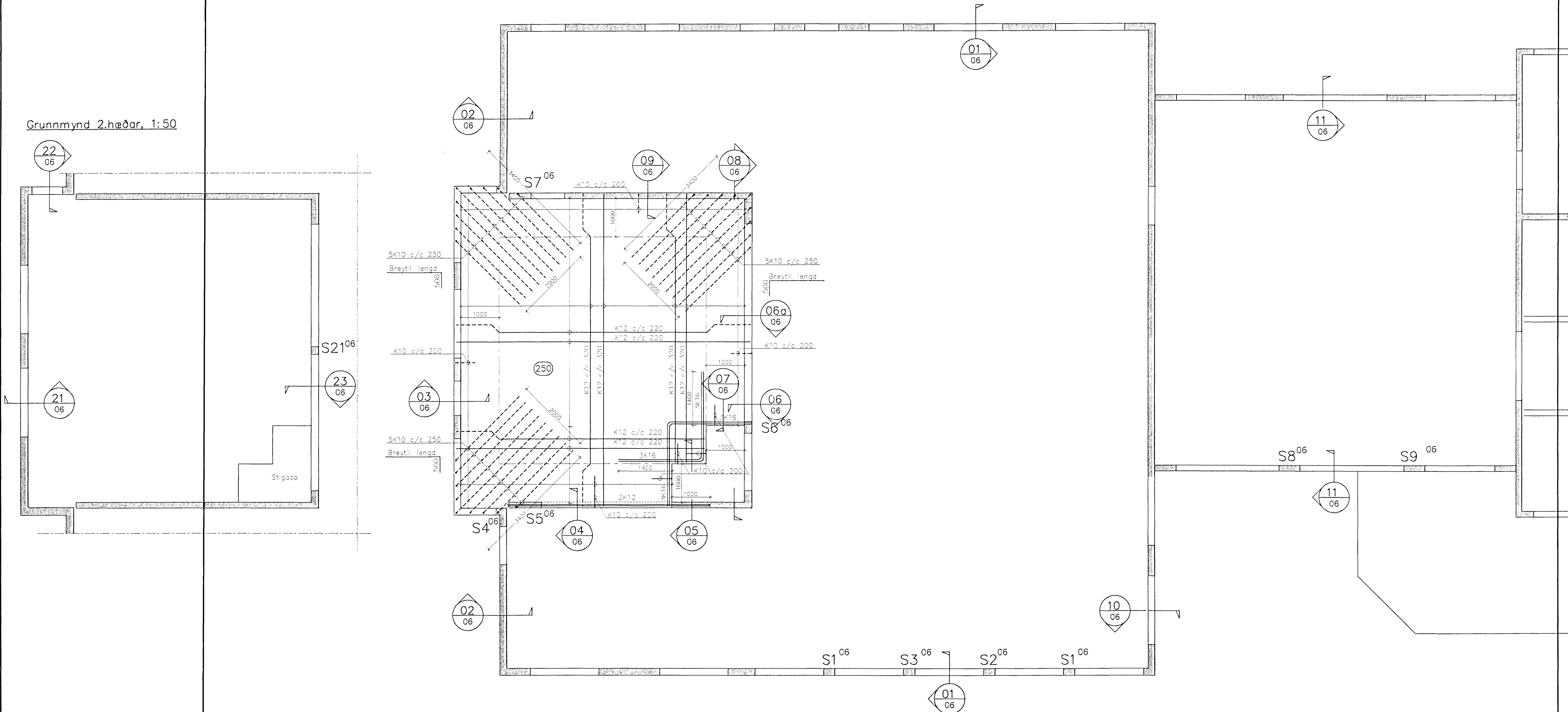
Grunnmynd 1.hæðar, 1:50
