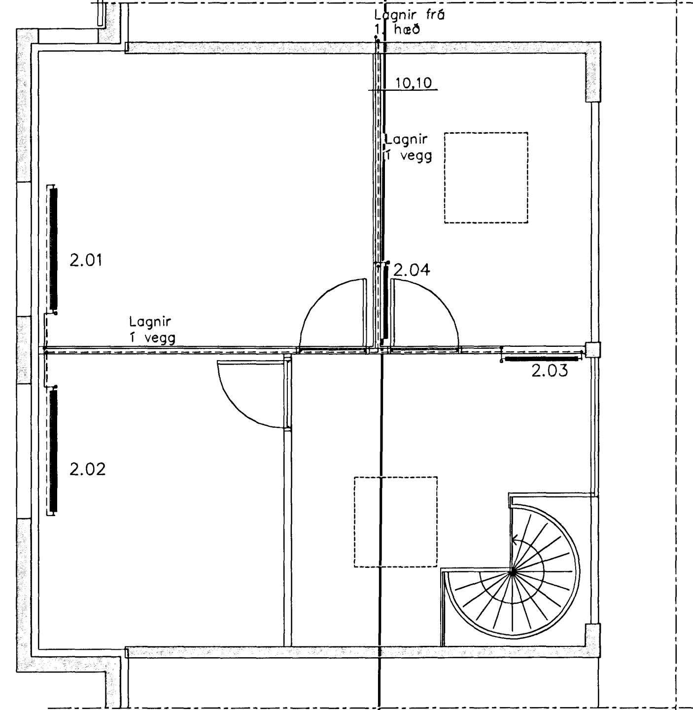
Grunnmynd 2.hæðar, 1:50
