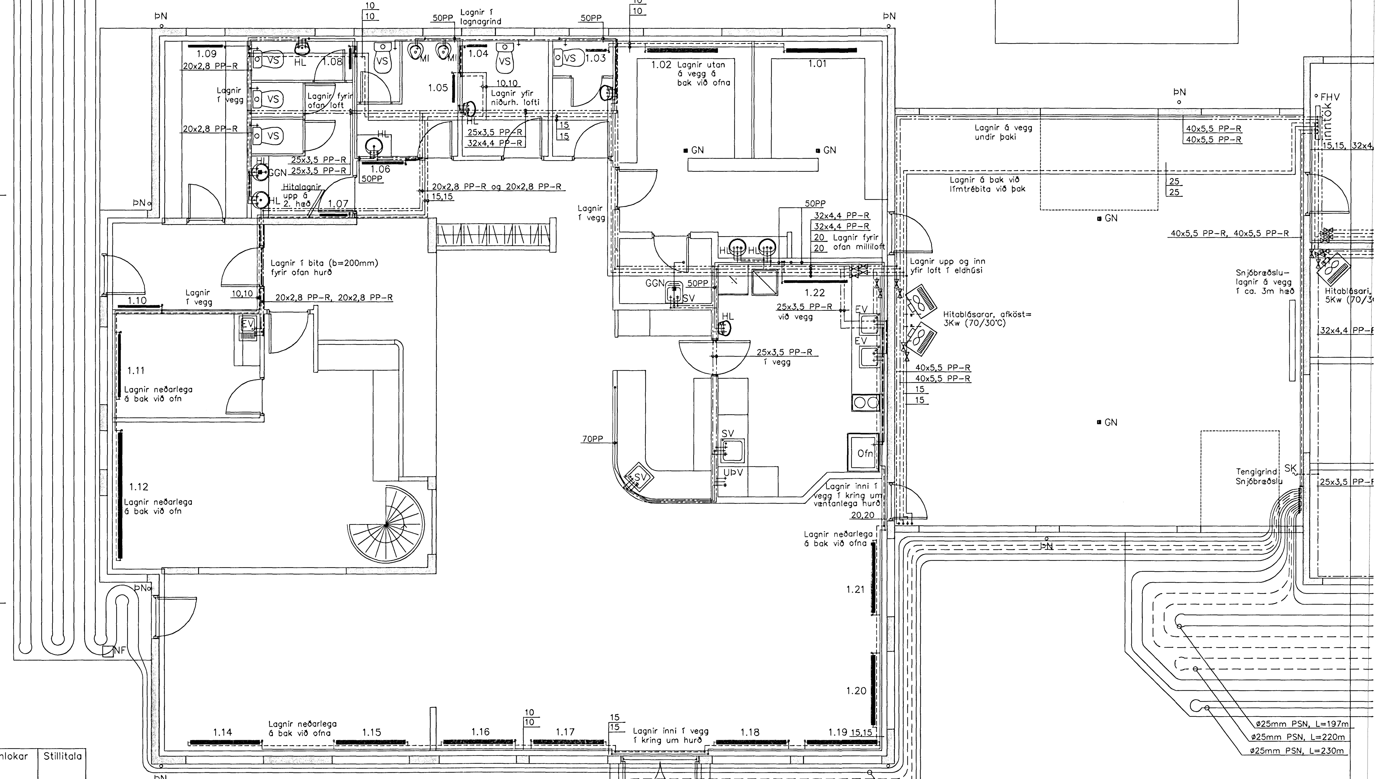
Grunnmynd 1.hæðar, 1:50
