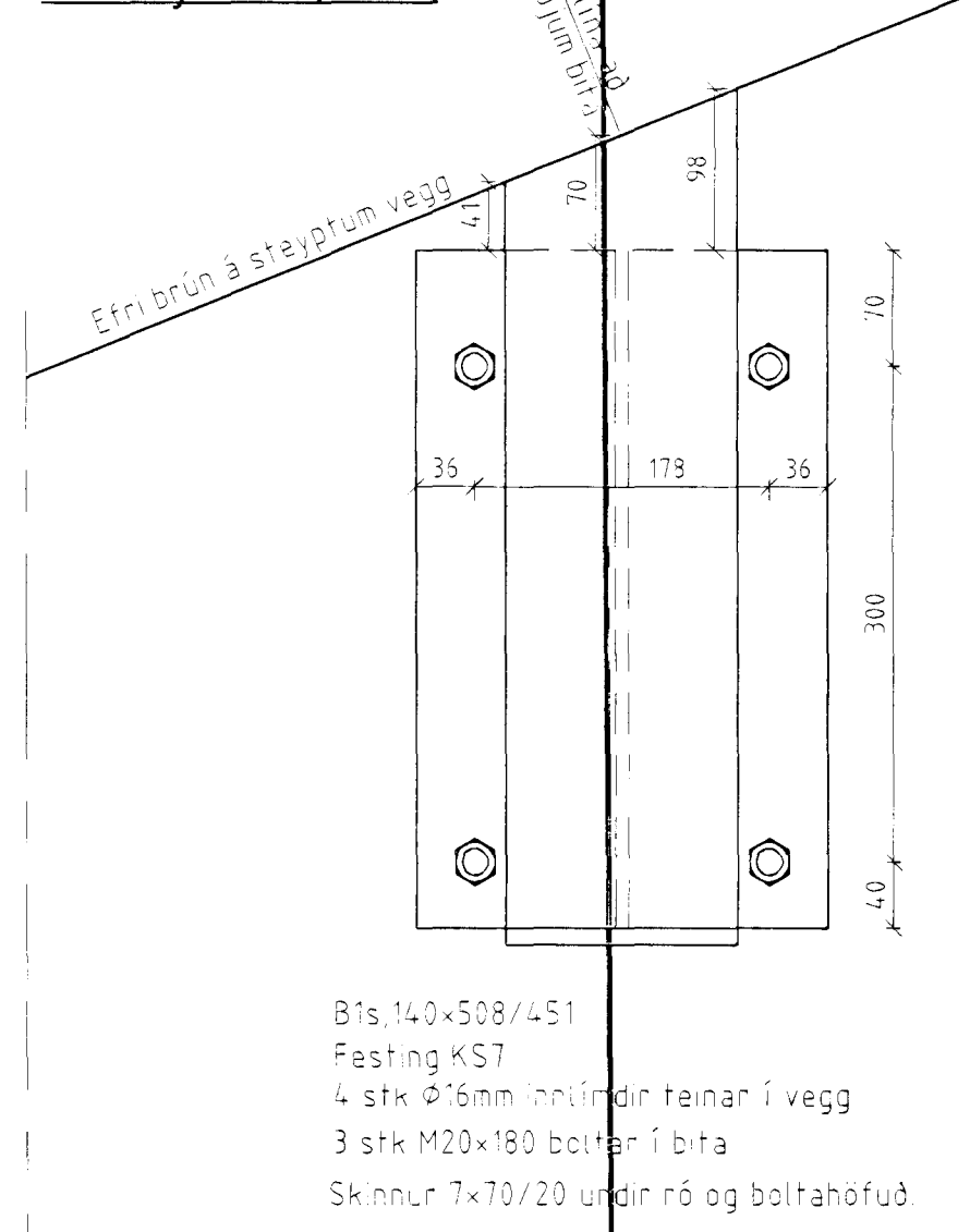
Sérmynd L, 1:5
