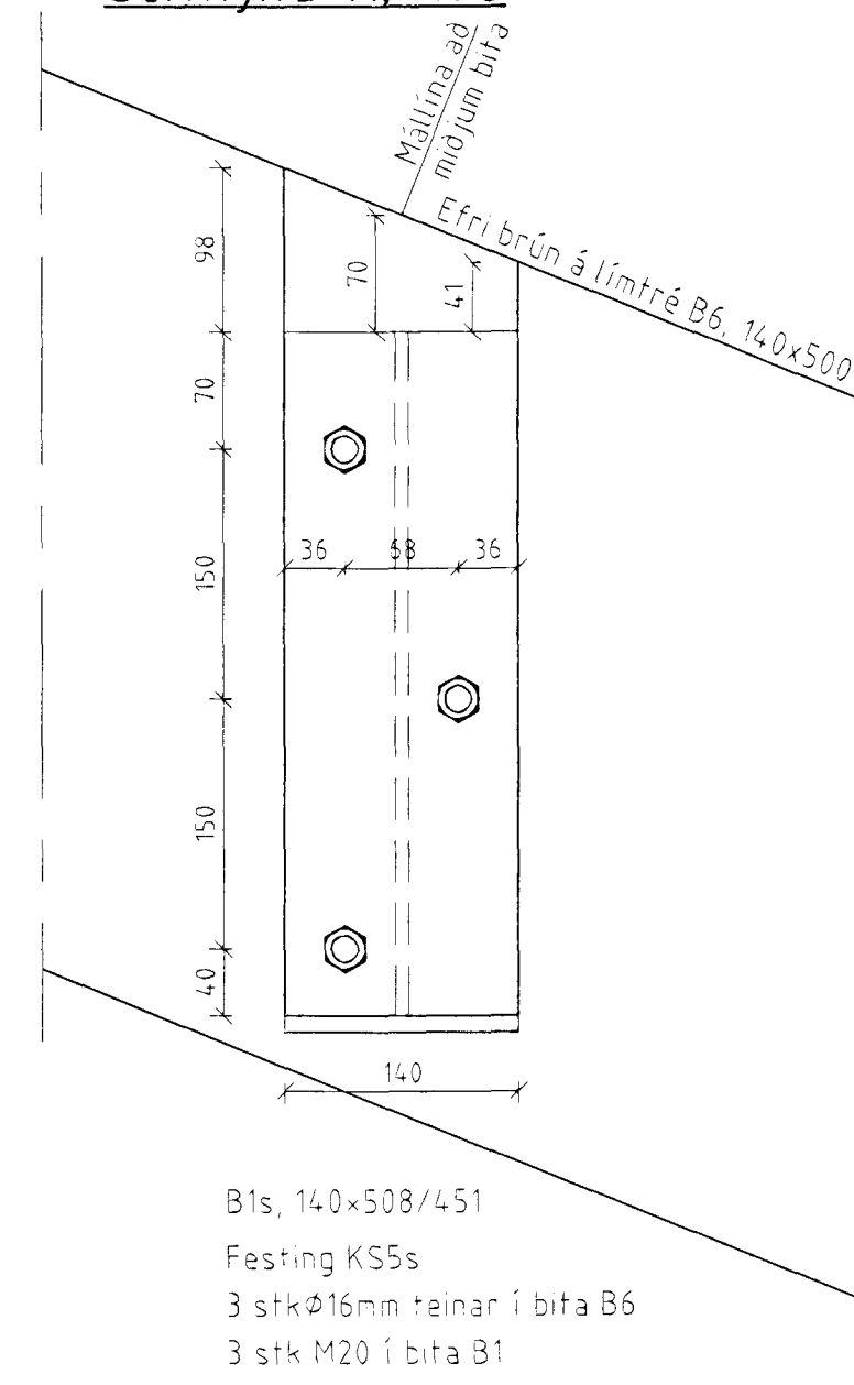
Sérmynd K, 1:5
