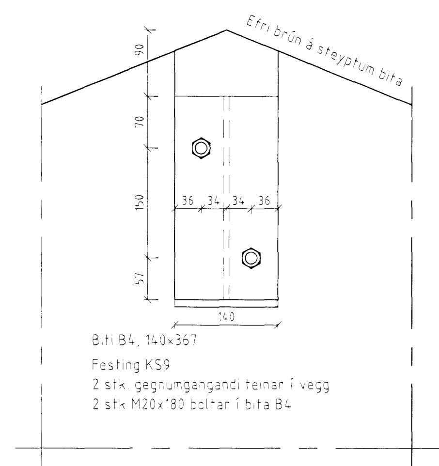
Sérmynd F, 1:5
