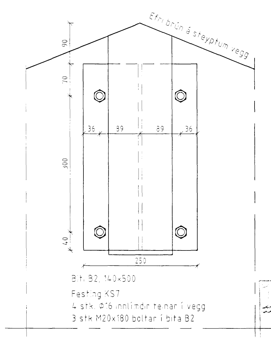
Sérmynd M, 1:5
