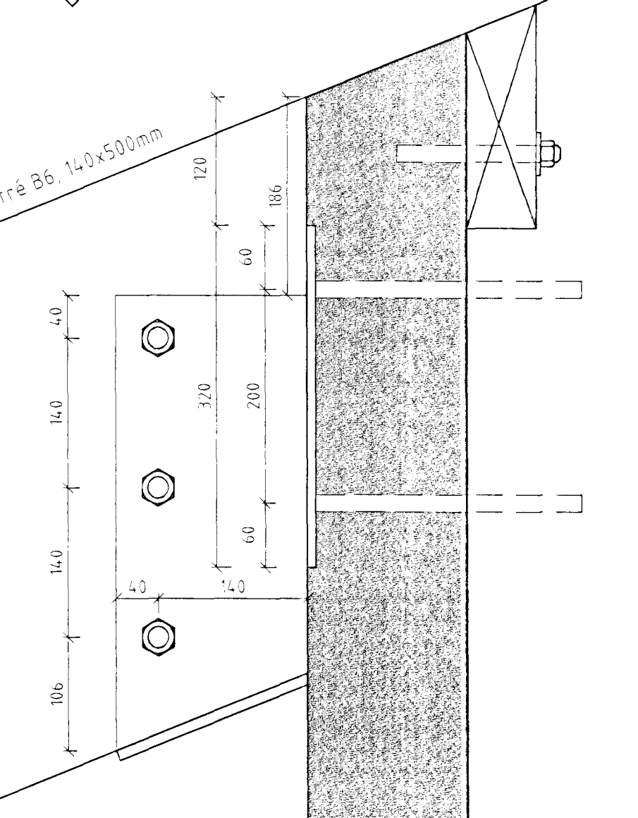
01 Snið, 1:5
