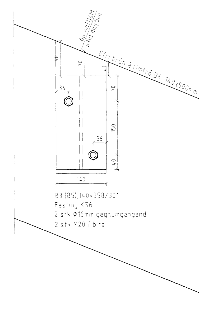
Sérmynd G, 1:5
