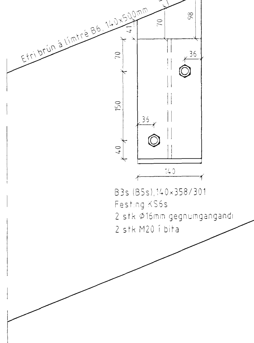
Sérmynd D, 1:5
