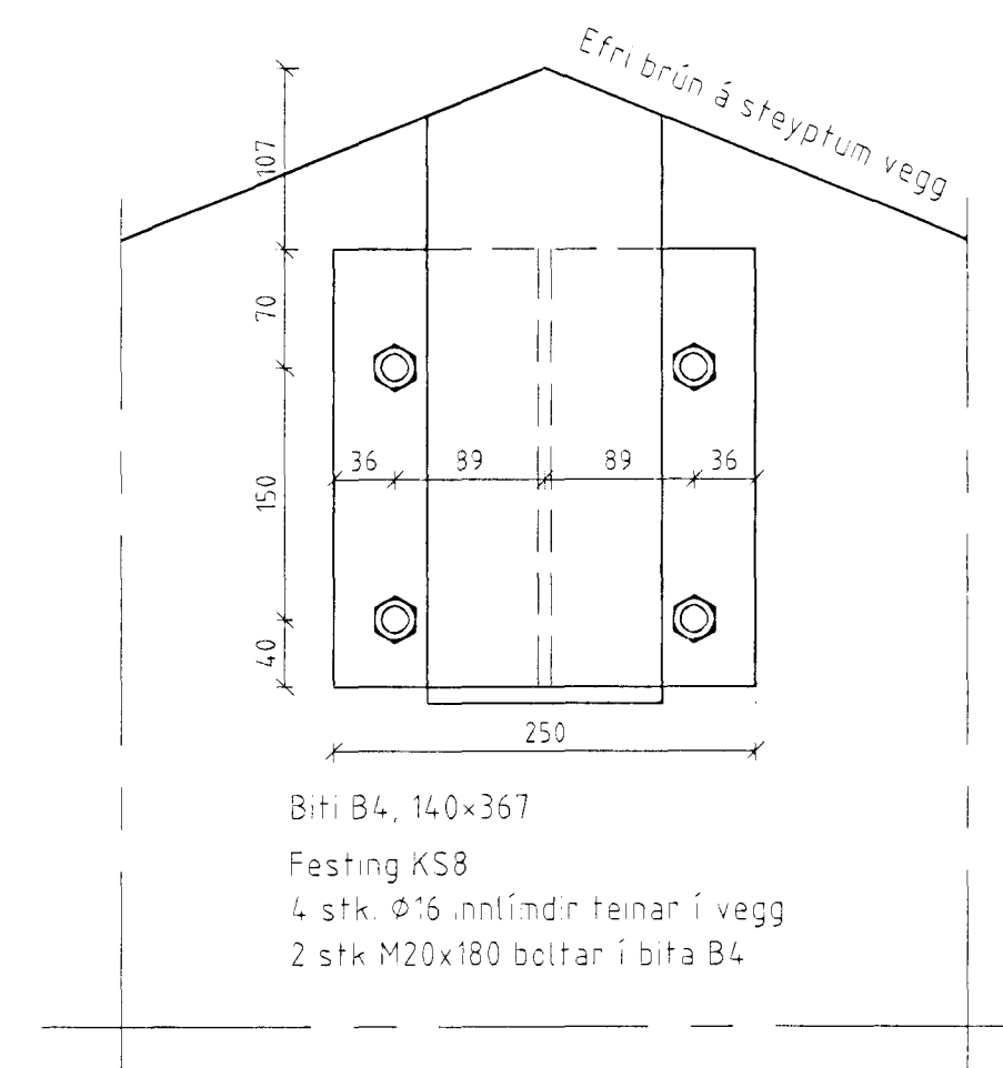
Sérmynd B, 1:5
