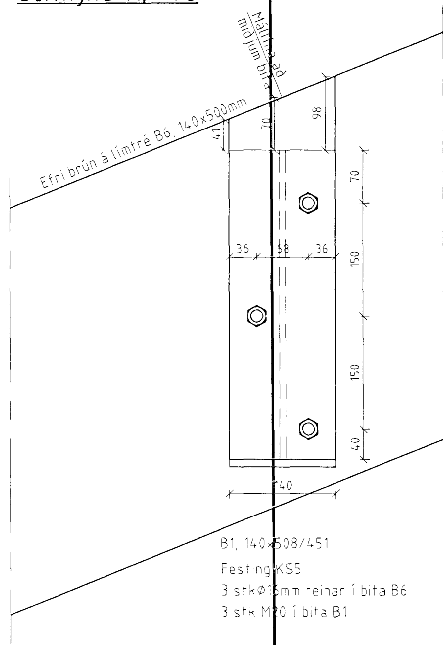
Sérmynd H, 1:5
