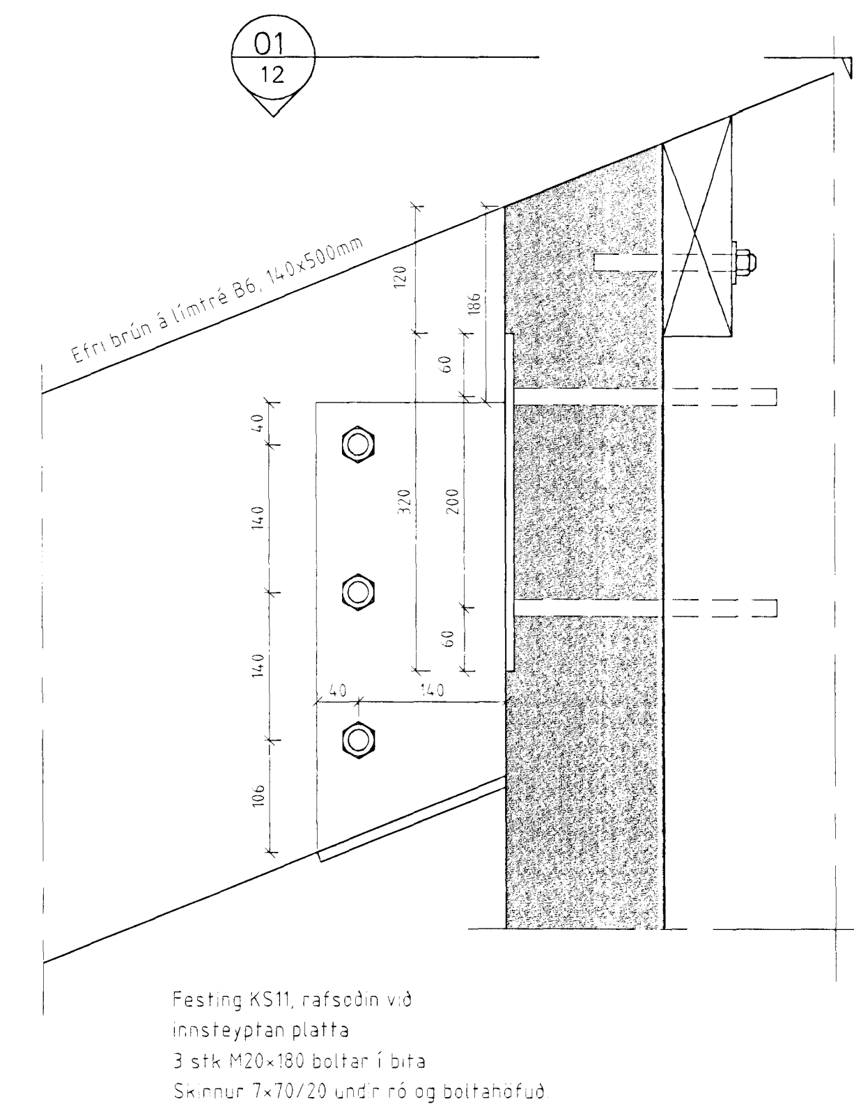
Sérmynd E, 1:5
