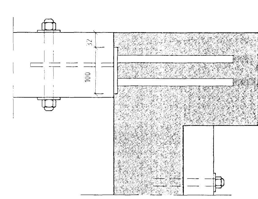
01 Snið, 1:5
