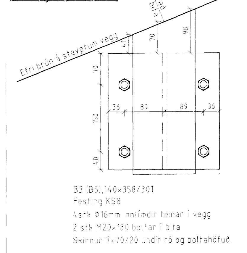
Sérmynd A, 1:5
