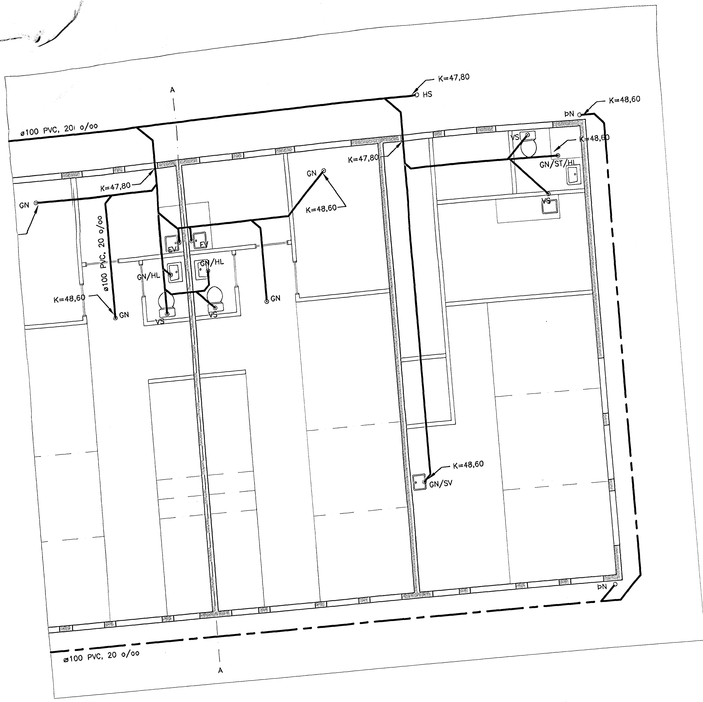
GRUNNMYND. 1:50
