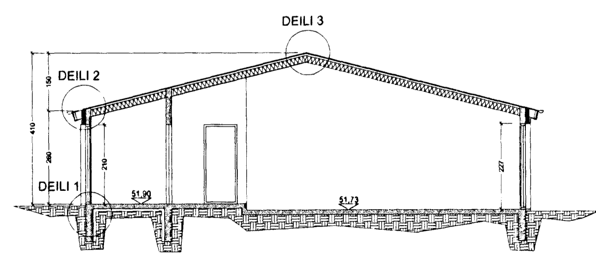
SKURÐUR A-A
