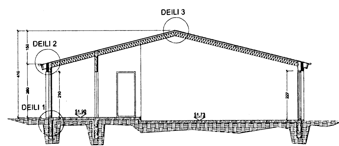
SKURÐUR A-A
