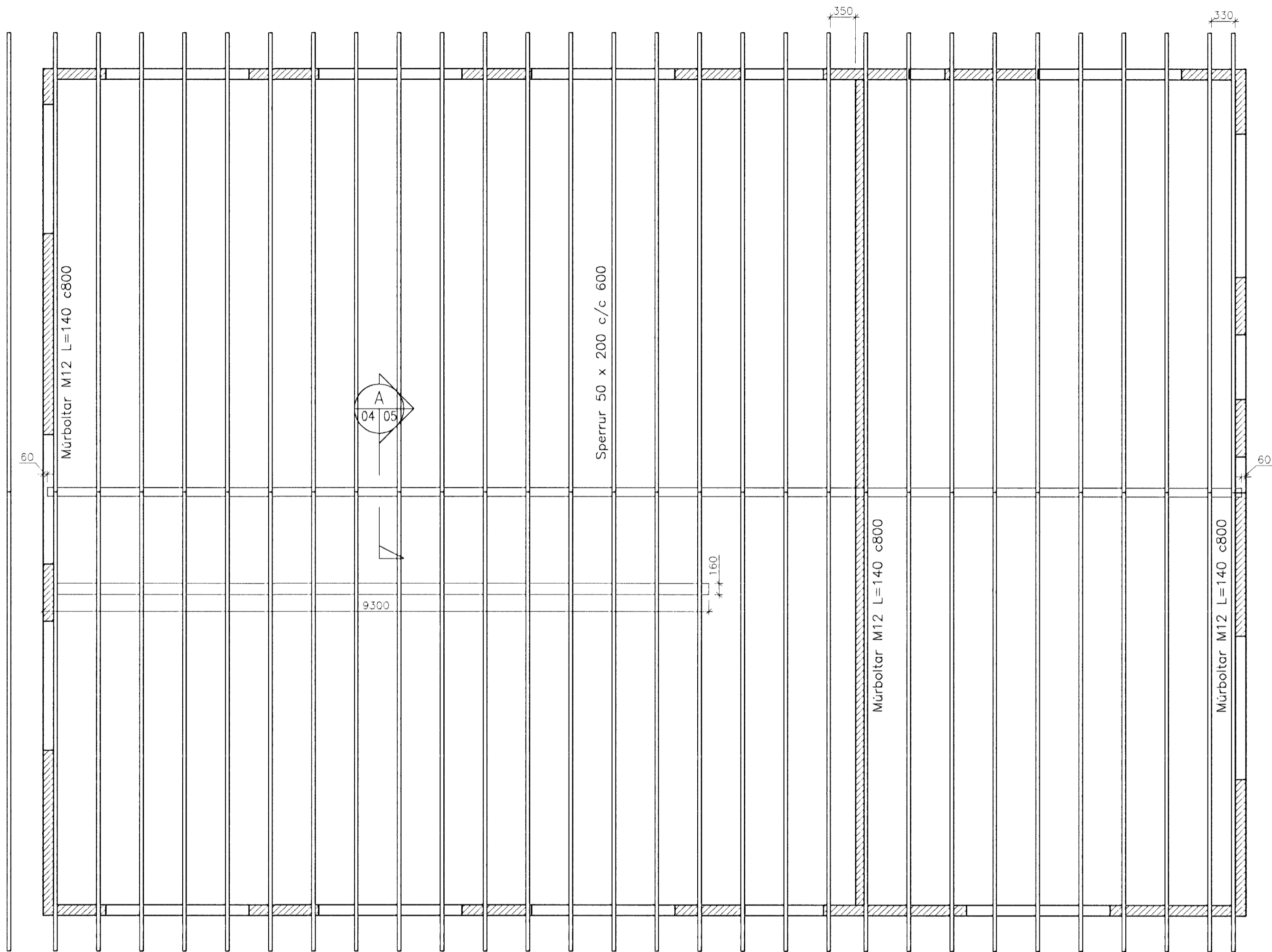
○ Grunnmynd Mkv. 1:50
