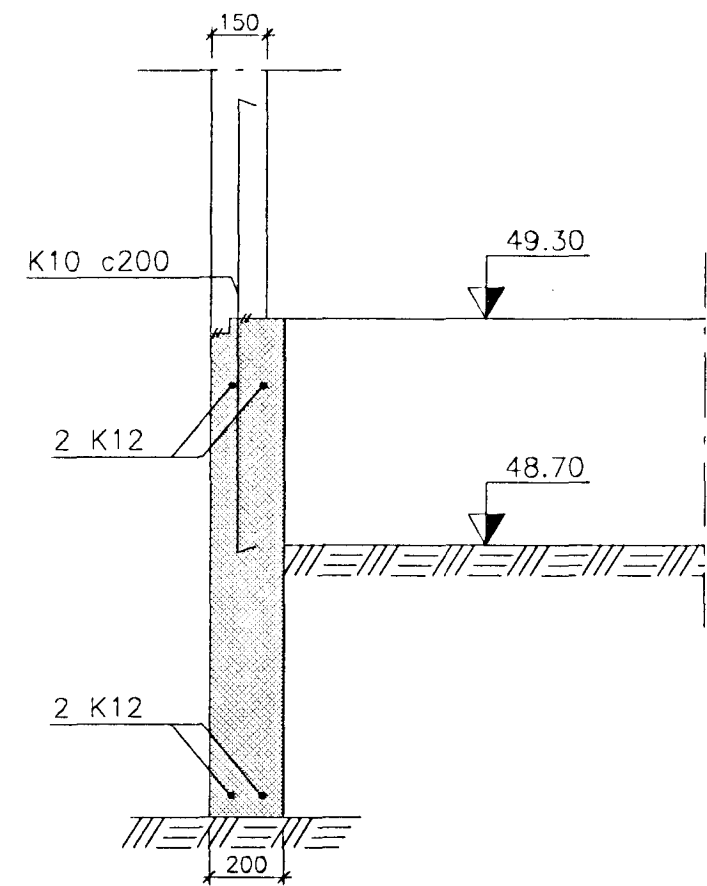
A Snið 02|03 Mkv. 1:20
