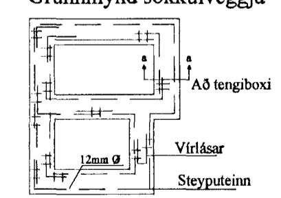
Grunnmynd sökkulvegga
