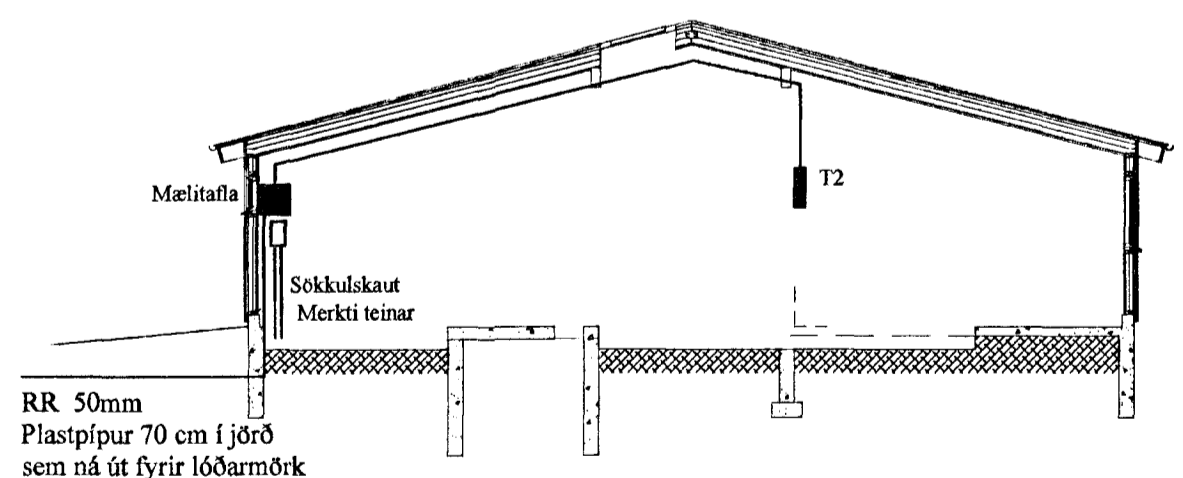
Snið a-a mkv. 1:100
