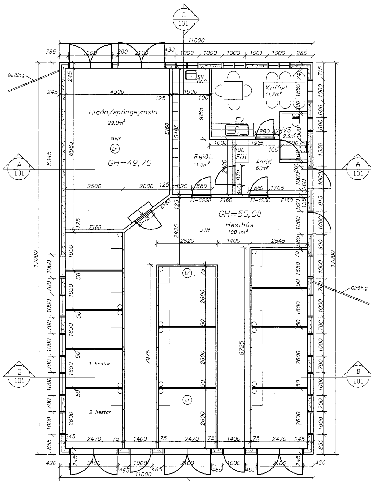
Grunnmynd
