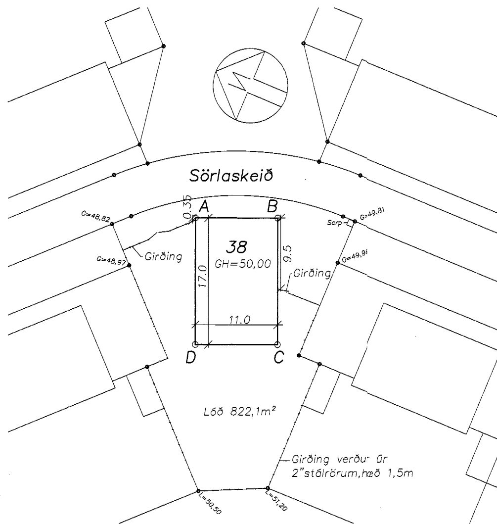
Afstaða 1:500
