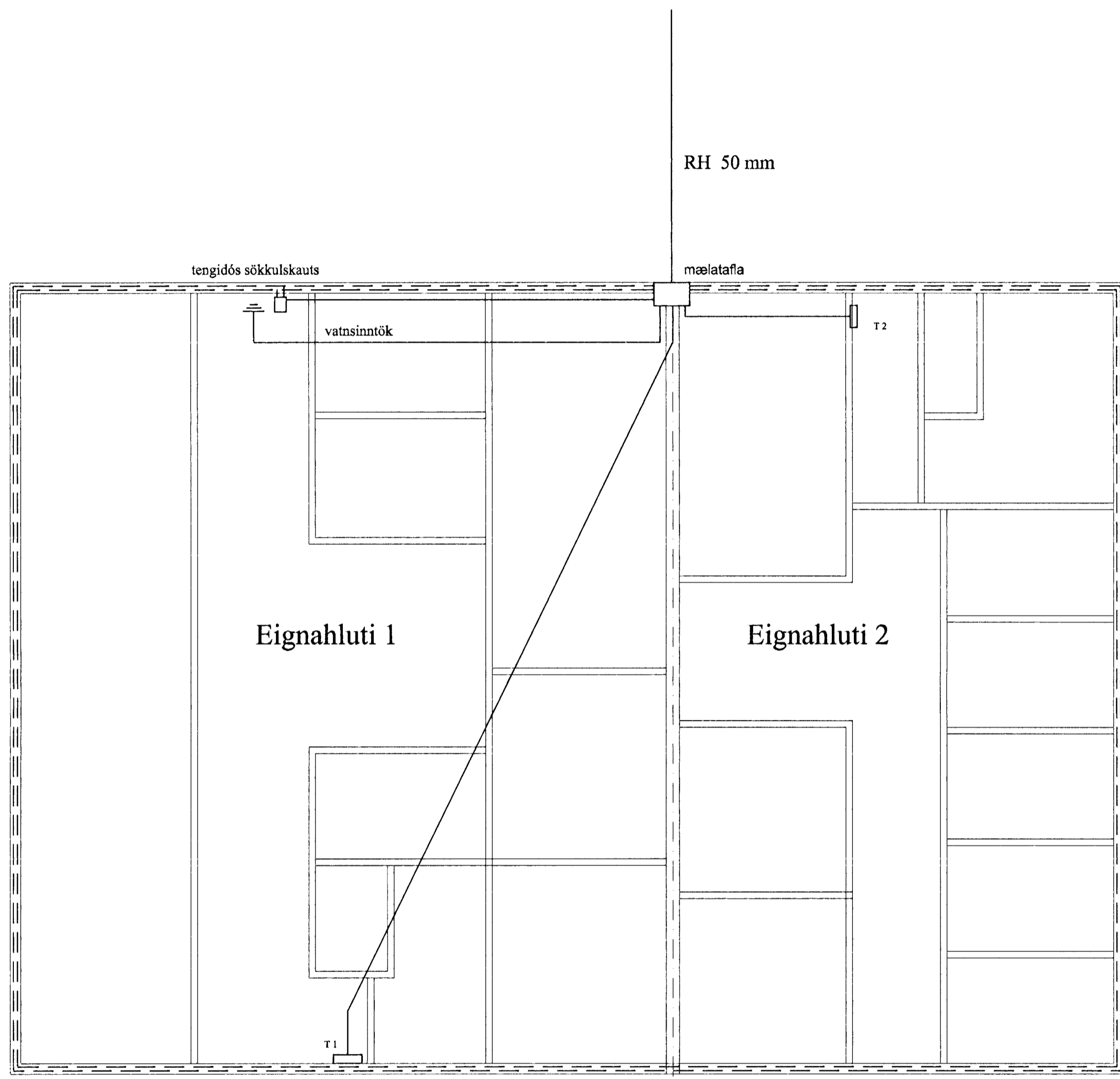
Grunnmynd sökkulskauts mkv.1:50
