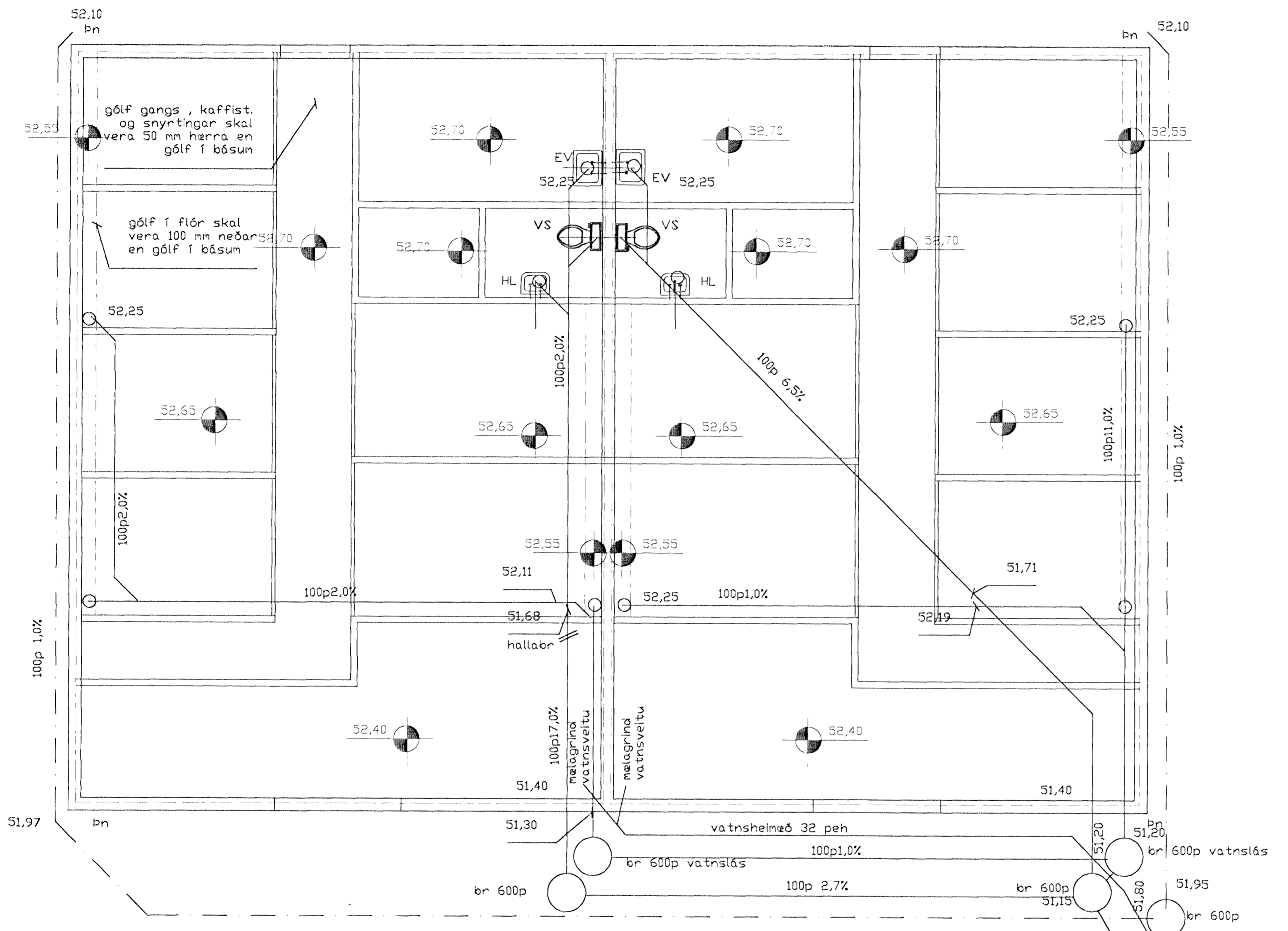
Grunnmynd grunnlagnir 1/50
