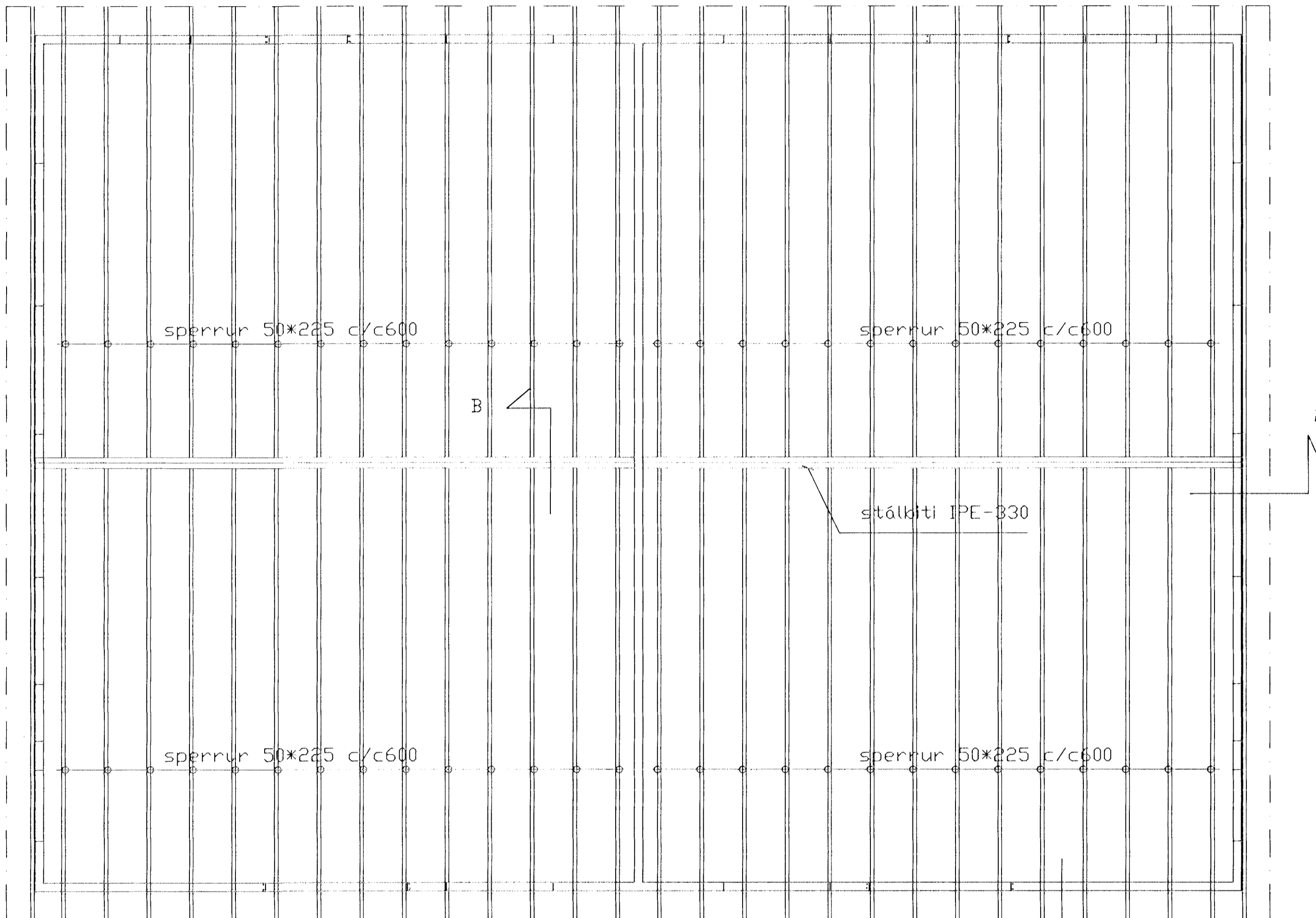
Grunnmynd 1/50
