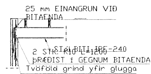
Snið 2, 1:20
