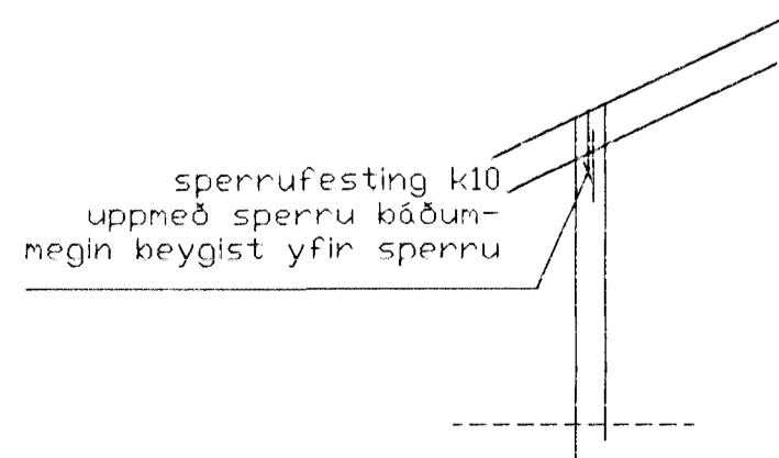
snið B 1/50
