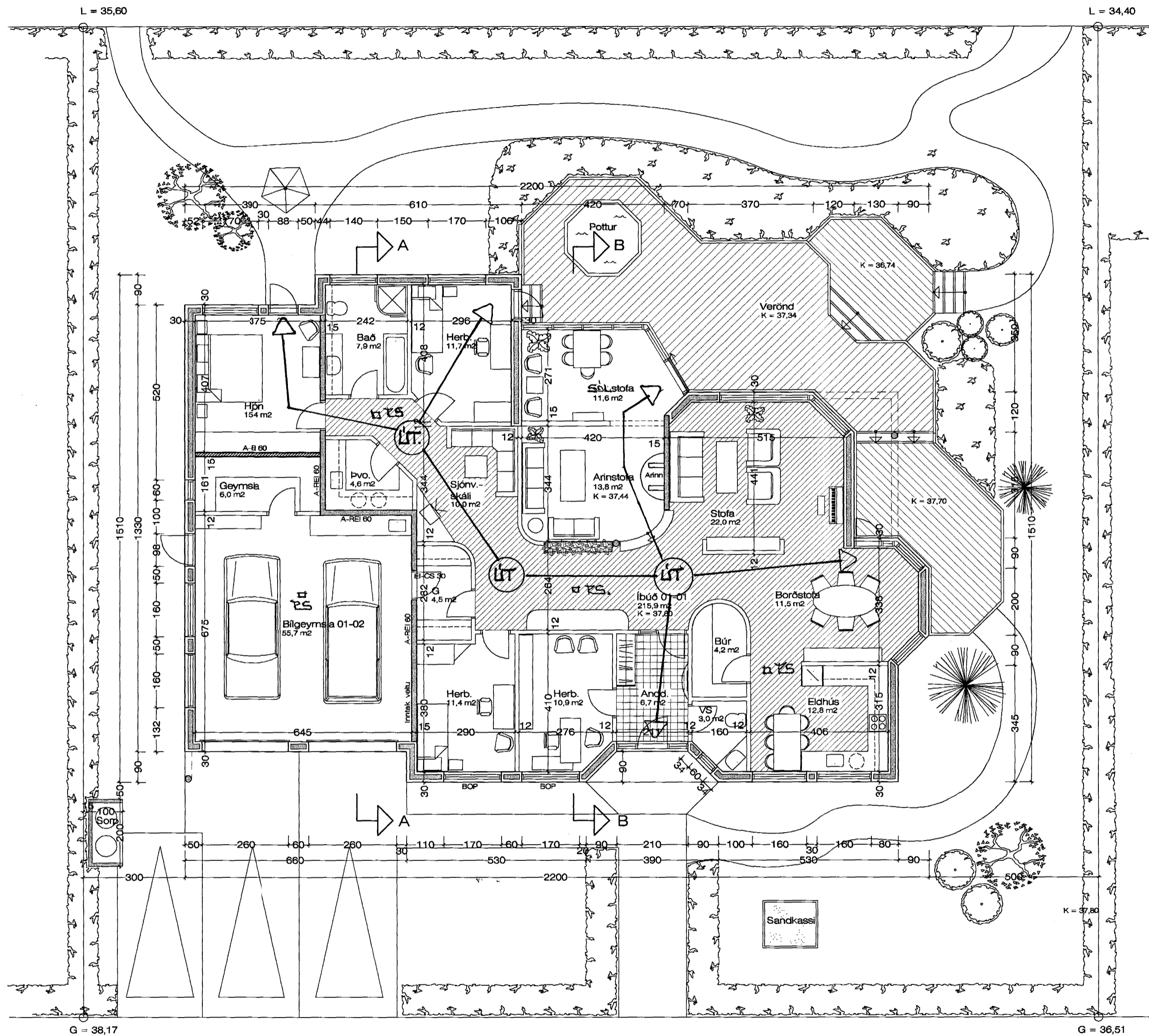
GRUNNMYND M 1 : 100
