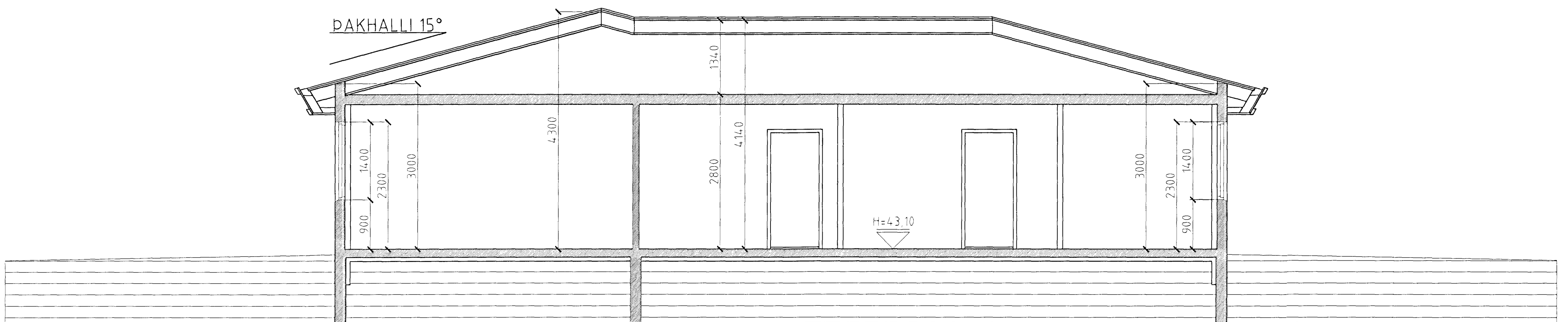
SNID B-B MKV. 1:50.
