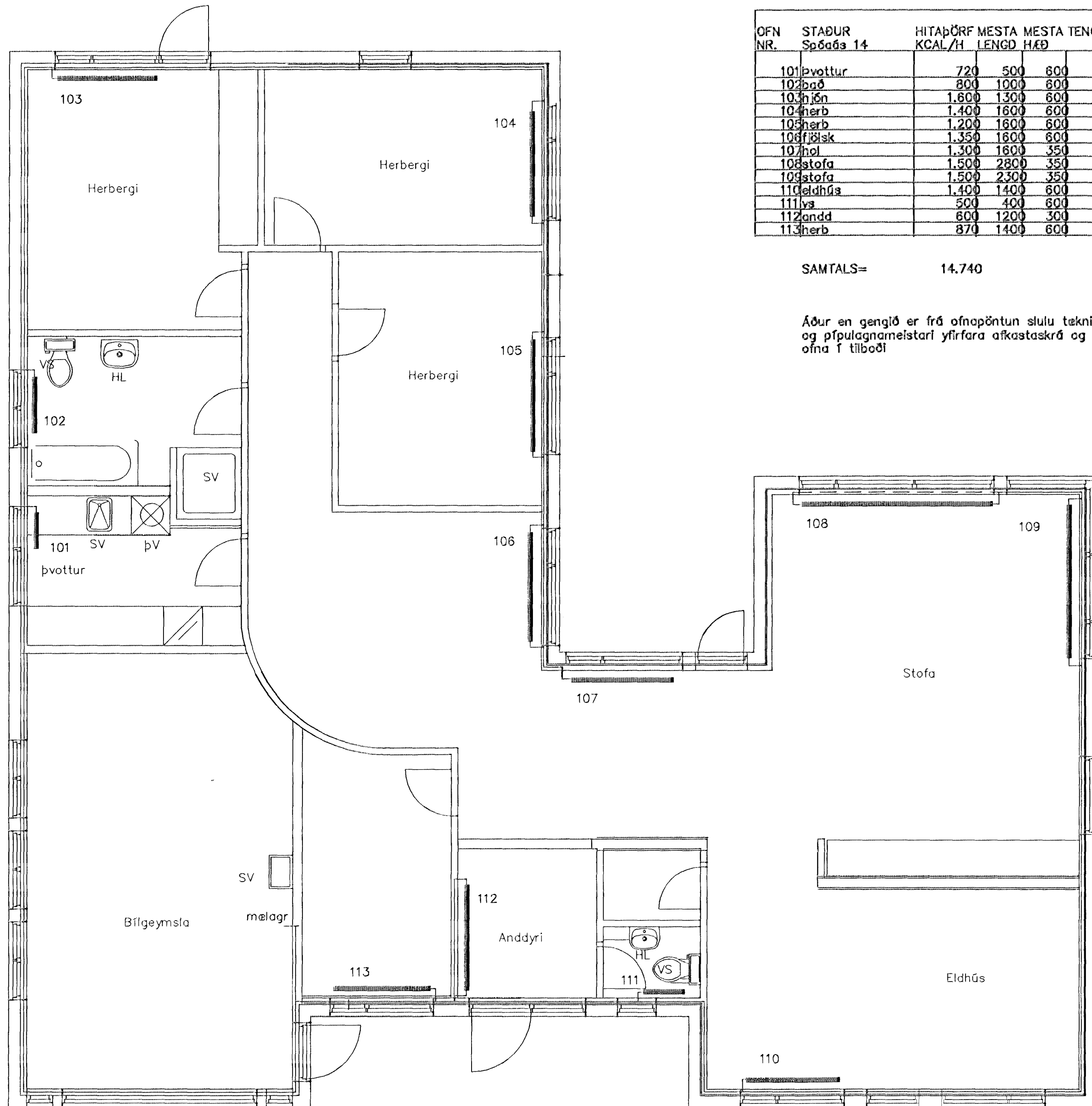
Grunnmynd 1:50
