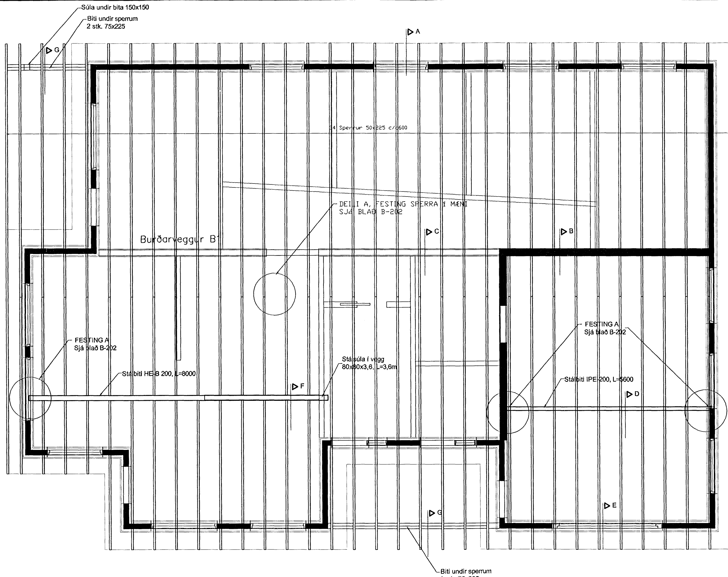
SPERRUPLAN, MKV. 1:50
