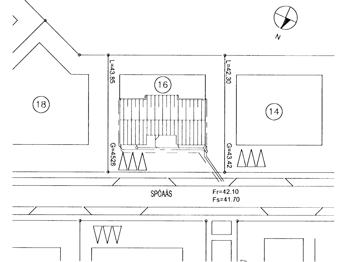
AFSTÖÐUMYND MKV. 1.500
