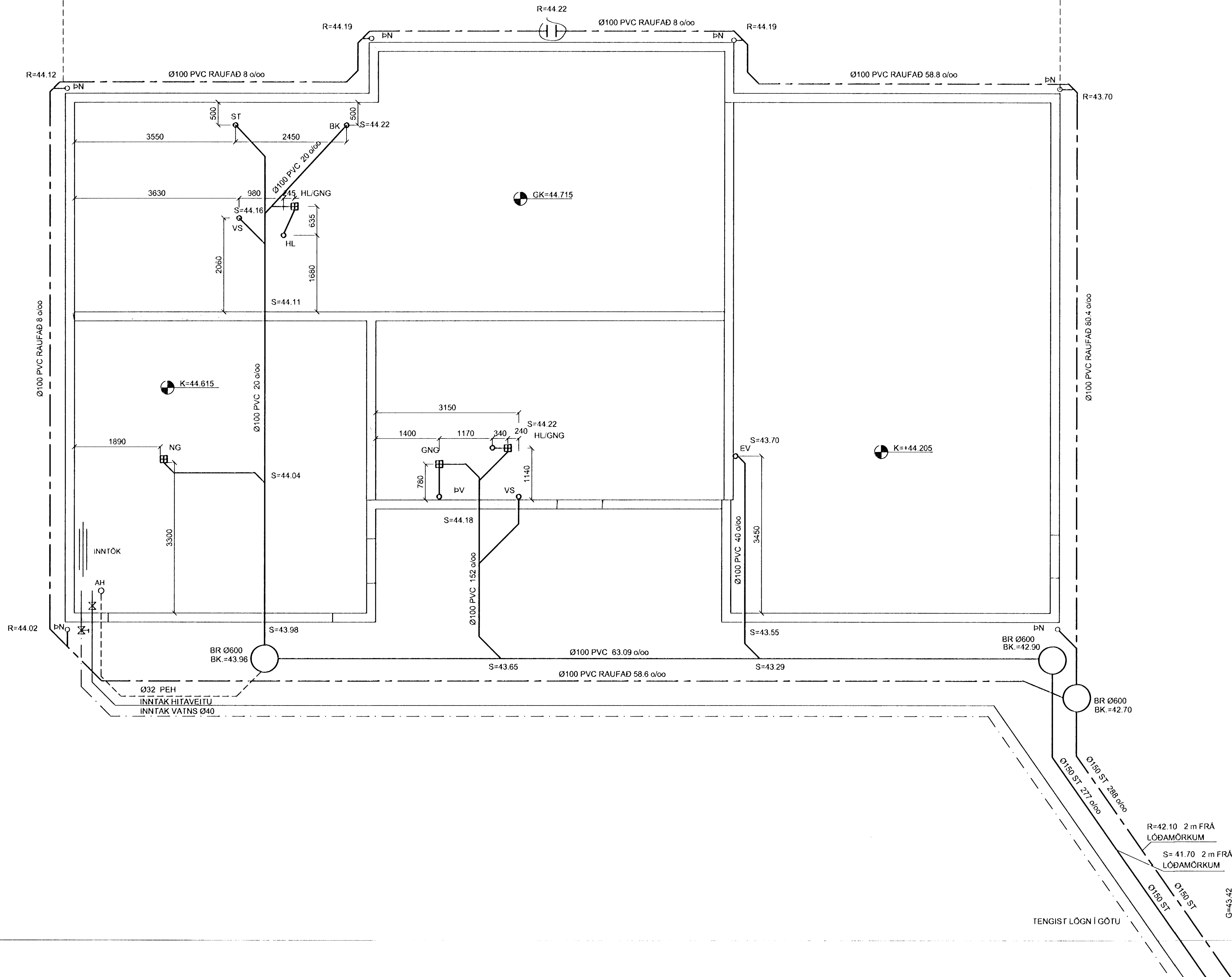
AFSTÖÐUMYND MKV. 1.500
