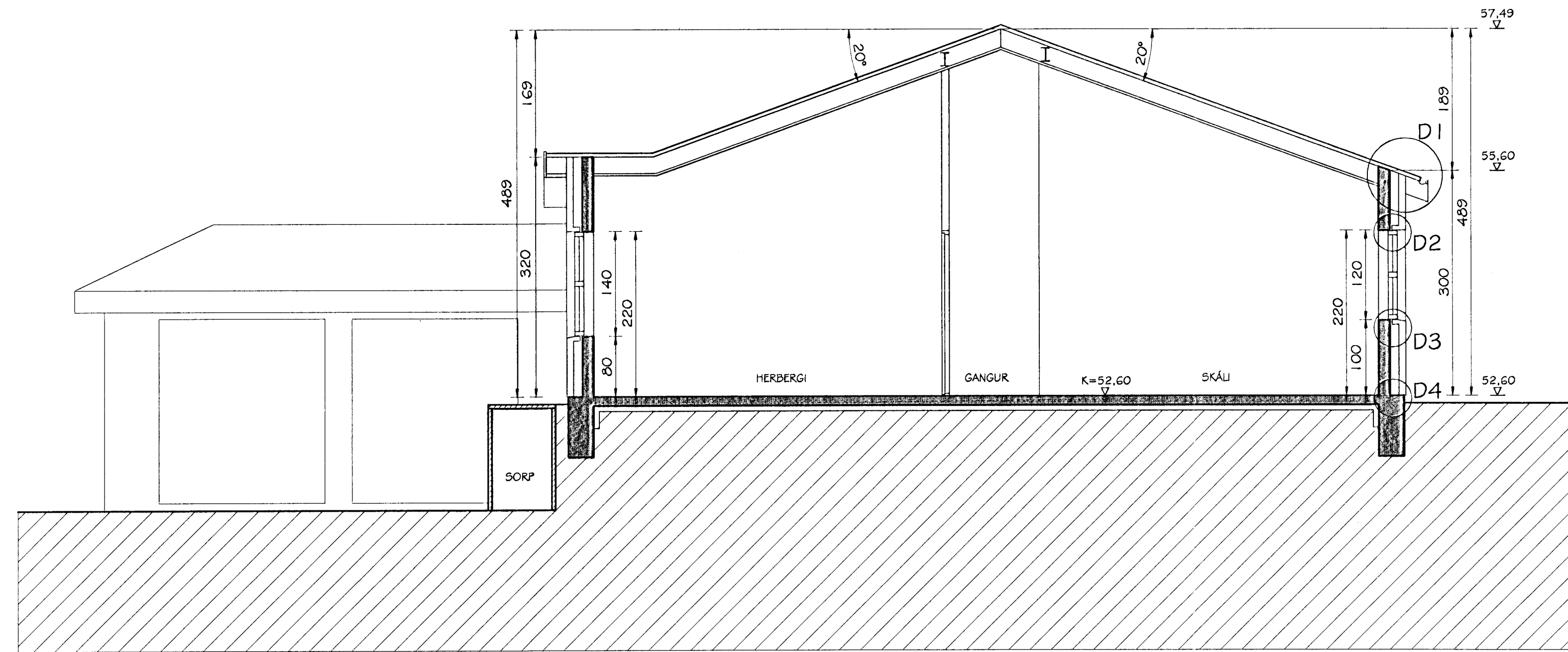
SNID C-C MKV. 1:50
