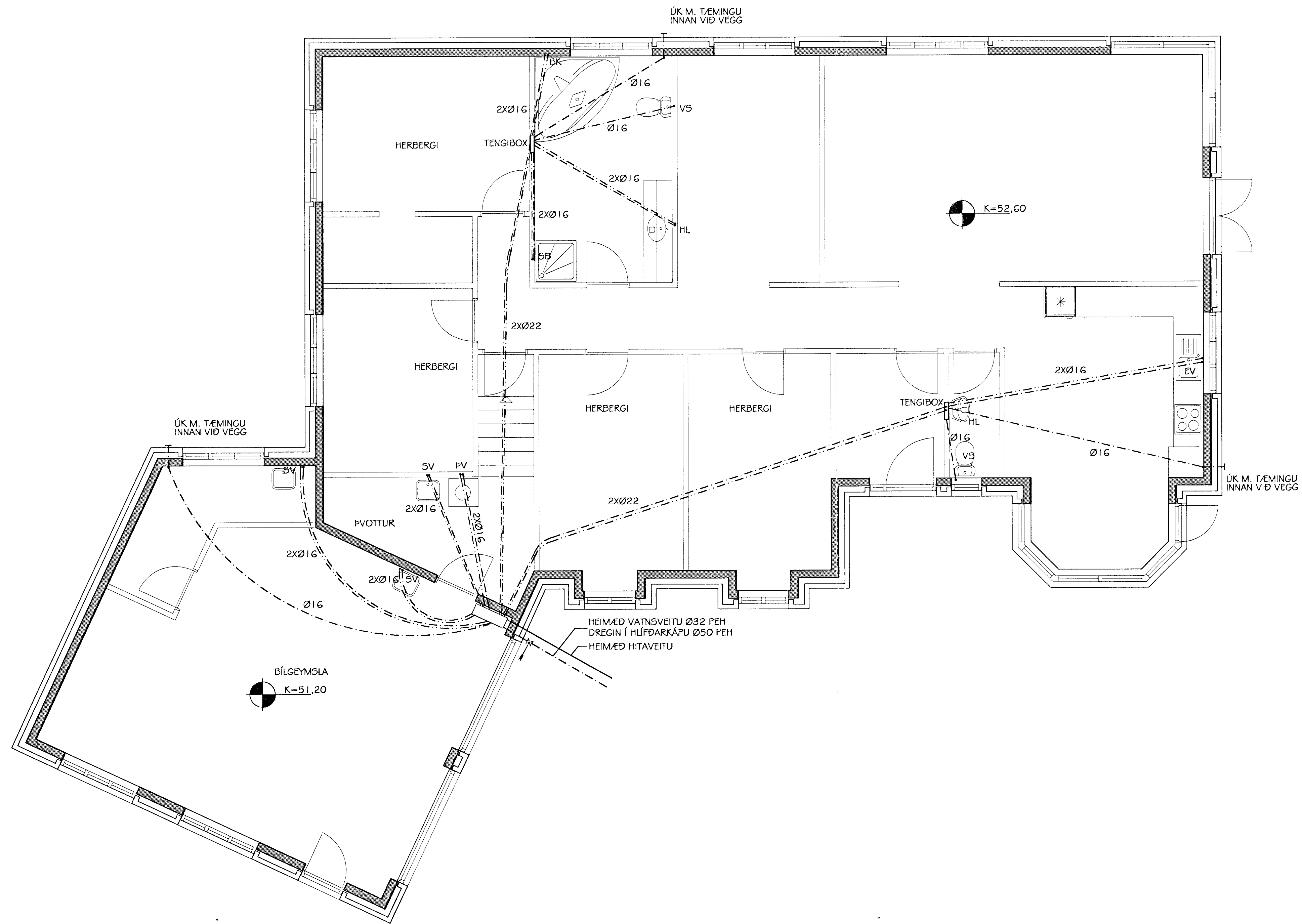
NEYSLUVATNSLAGNIR - GRUNNMYND MKV. 1:50
