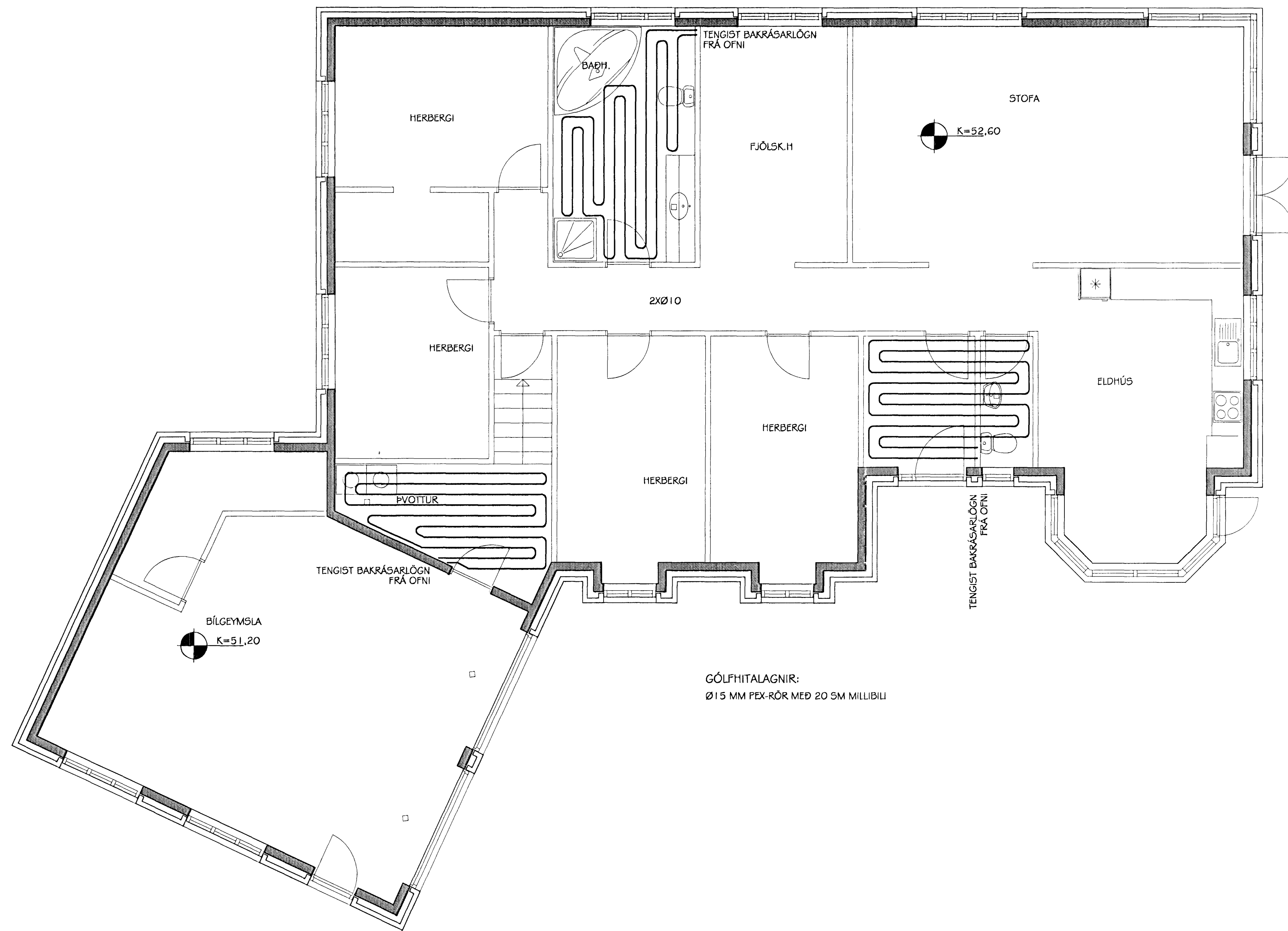
GÓLFHITALAGNIR - GRUNNMYND MKV. 1:50
