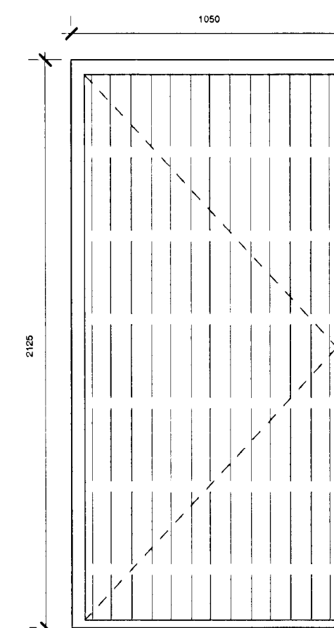
ÚH 4 ÍSTEYPTUR KARMUR 1 STK. HURÐ EKKI MEDTALIN
