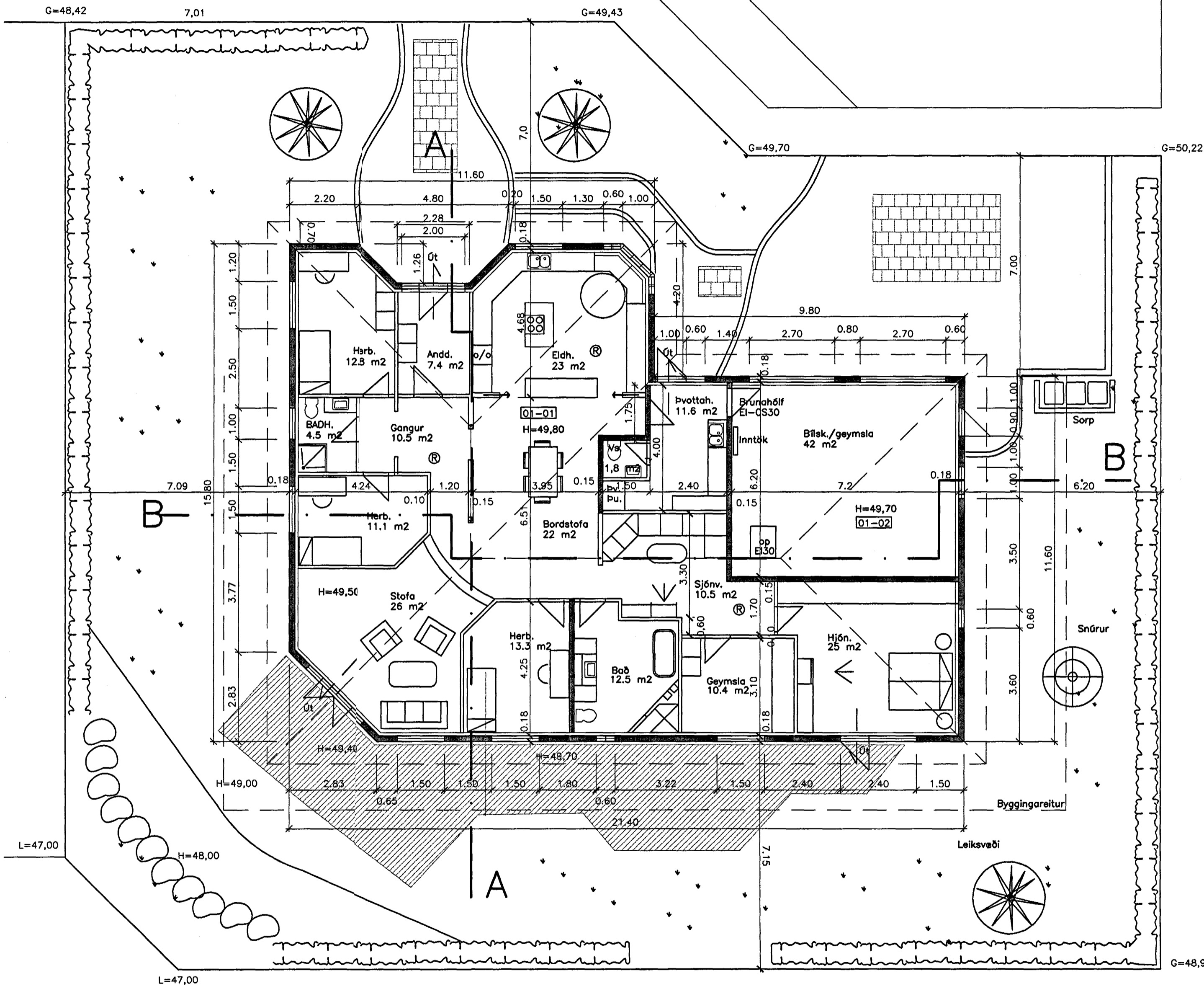
HÆÐ, GRUNNMYND
