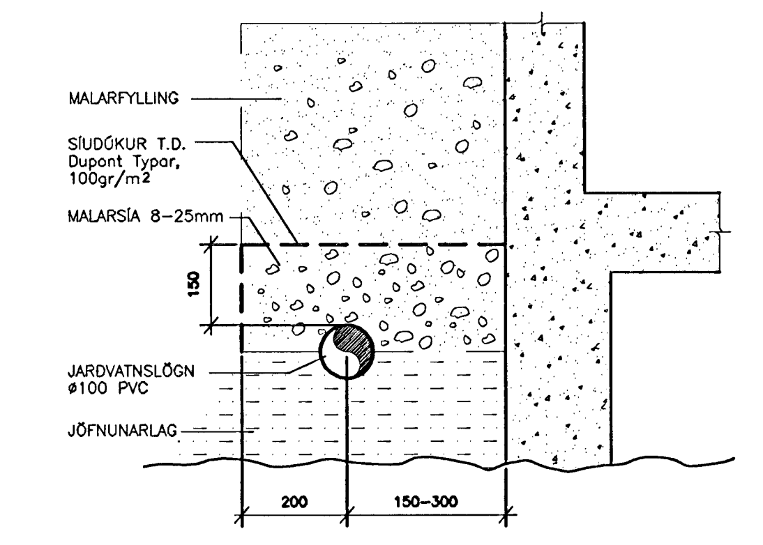
FRÁGANGUR JARÐVATNSLAGNA ÚR PVC M=1:20
