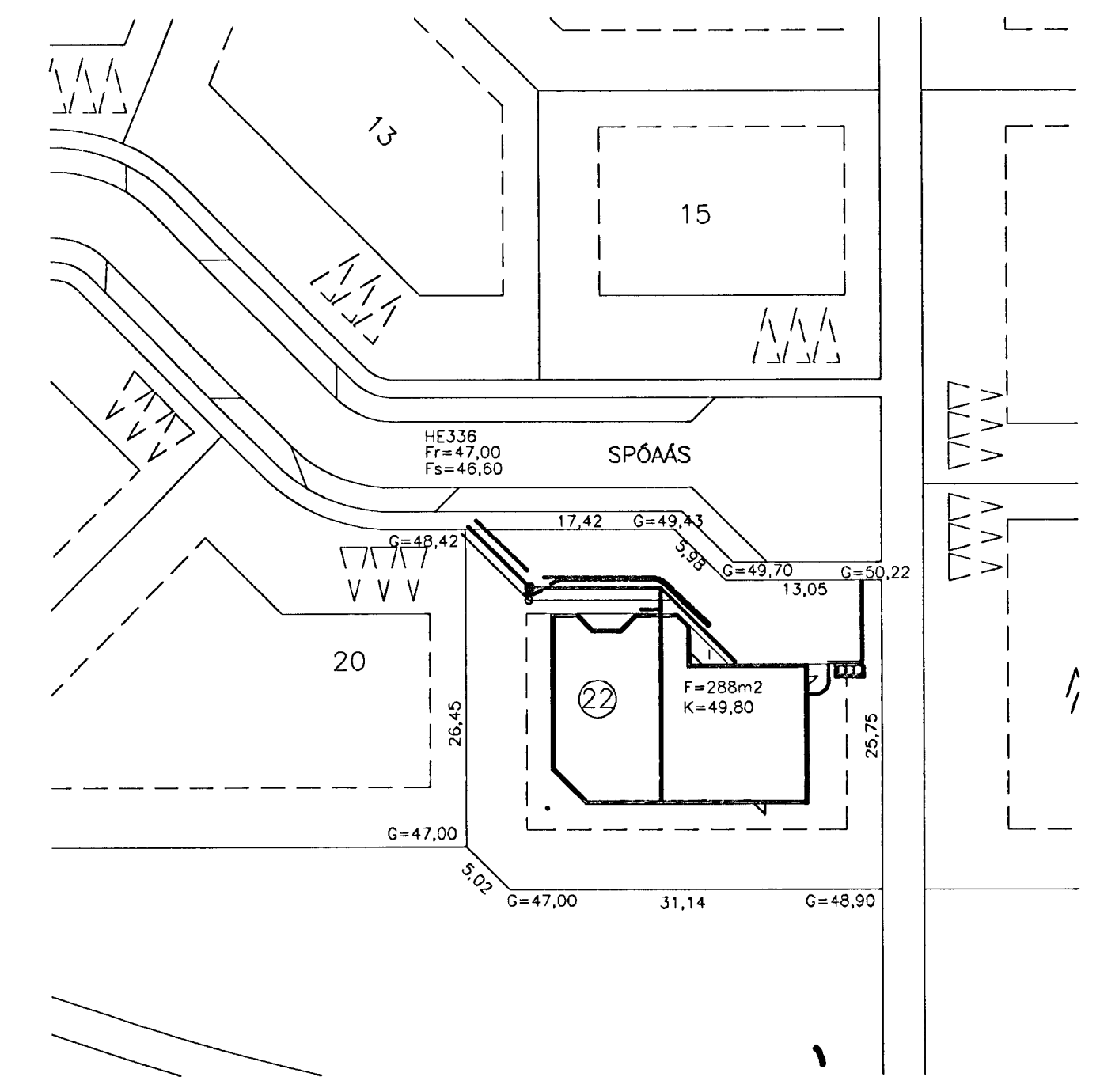
AFSTÖÐUMYND 1:50
