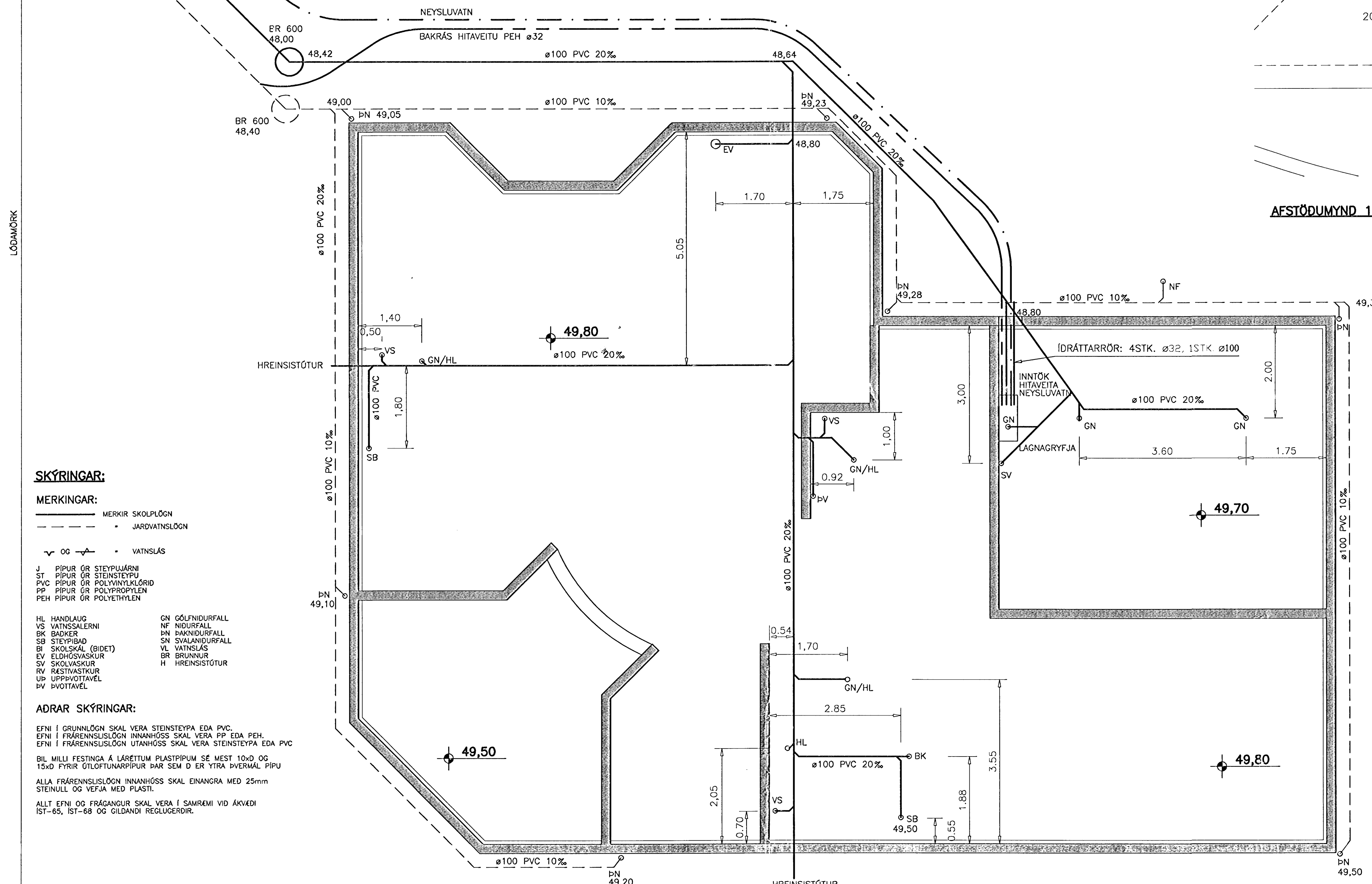
GRUNNMYND 1:50
