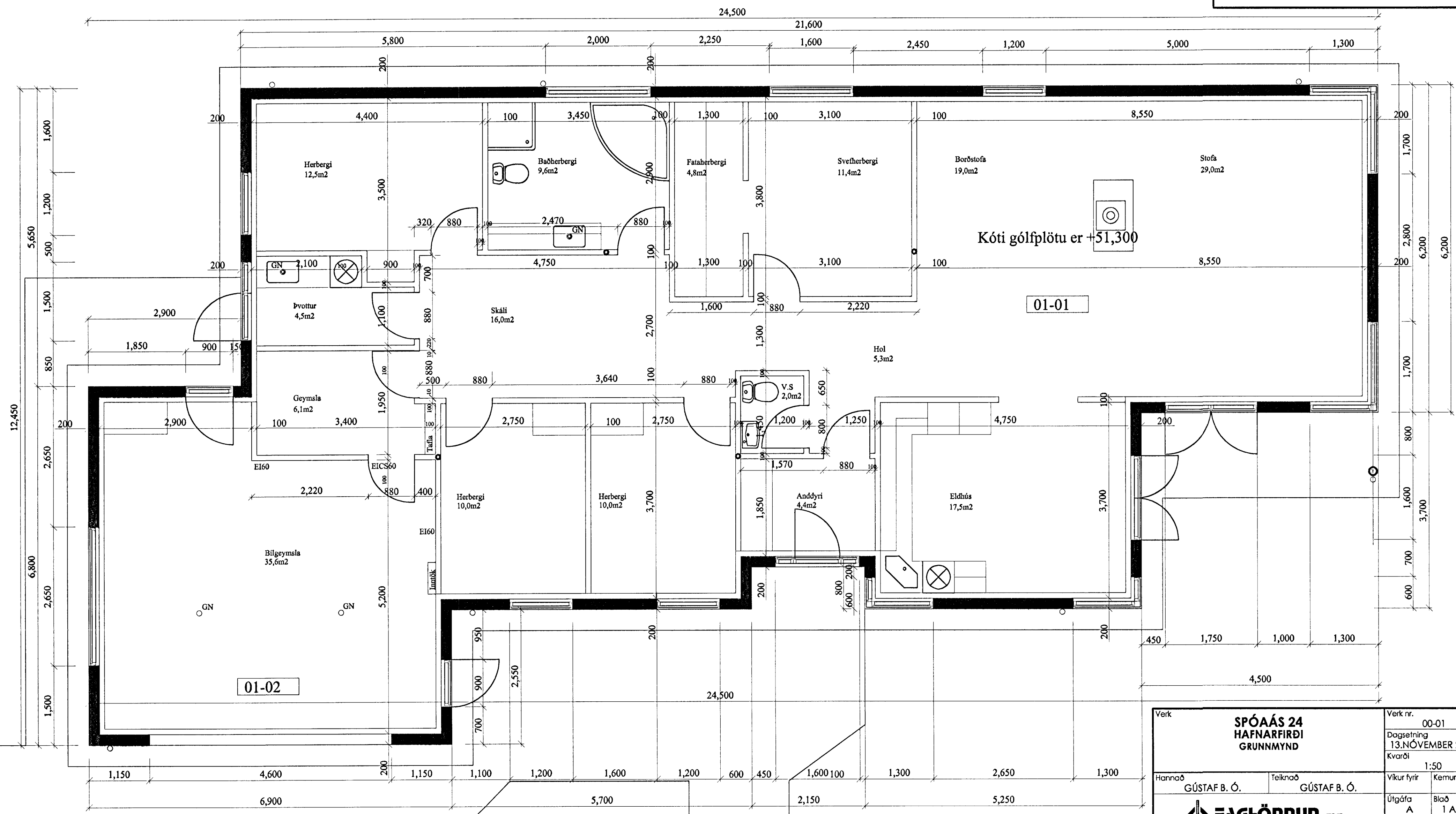
Grunnmynd mkv. 1:50
