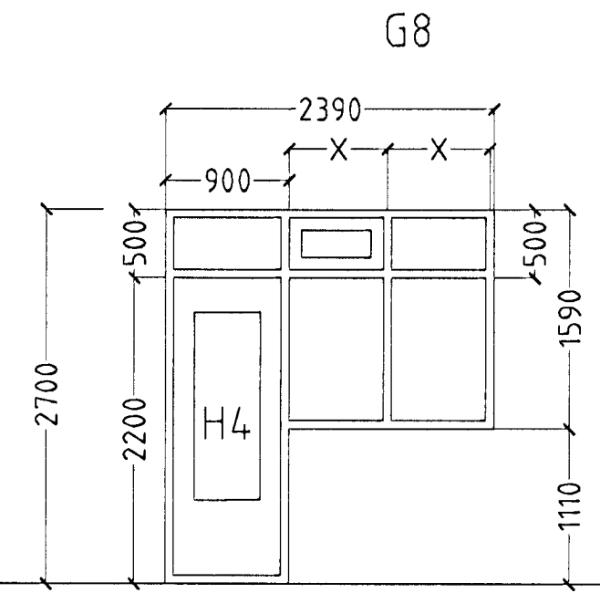
1 STK. FJÖLSKYLDA. HURÐ OPNAST VINSTRI ÚT.
