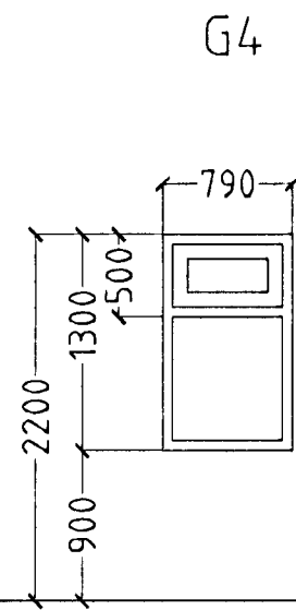
1 STK. ELDHÚS.
