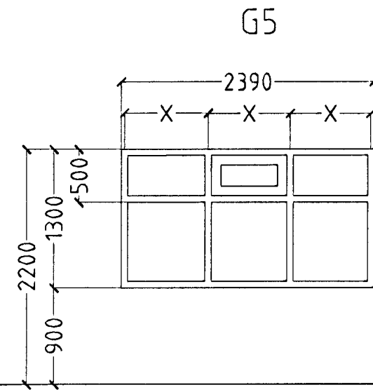
1 STK. BORBSTOFA.
