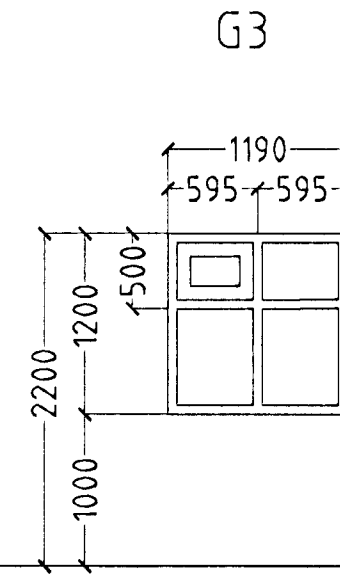
3 STK. ELDHÚS.
