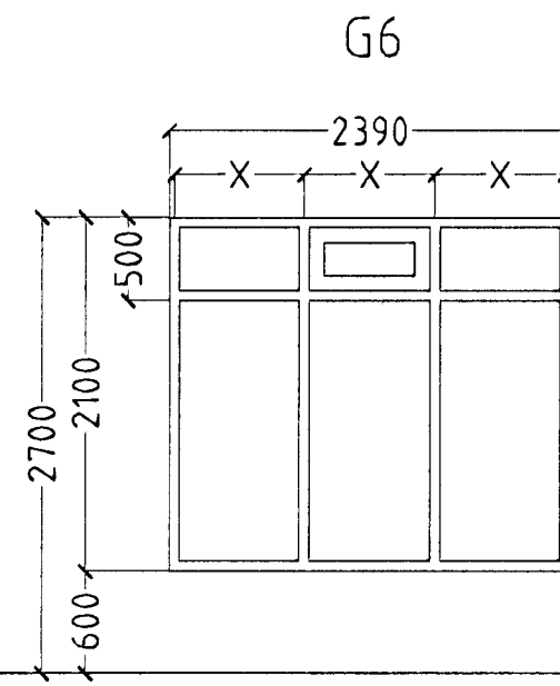
2 STK. STOFA.
