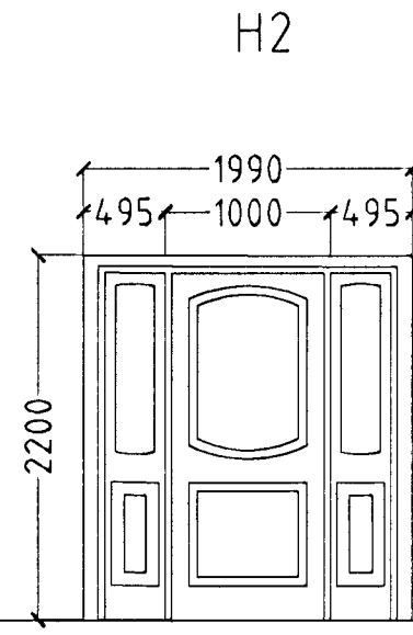
1 STK. ANDDYRISHURÐ. HURÐ OPNAST HÆGRI ÚT.
