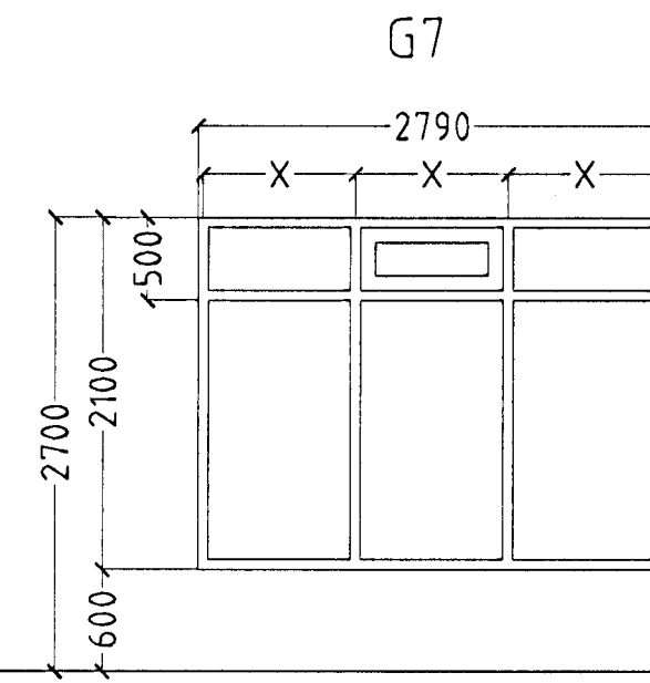
1 STK. STOFA.
