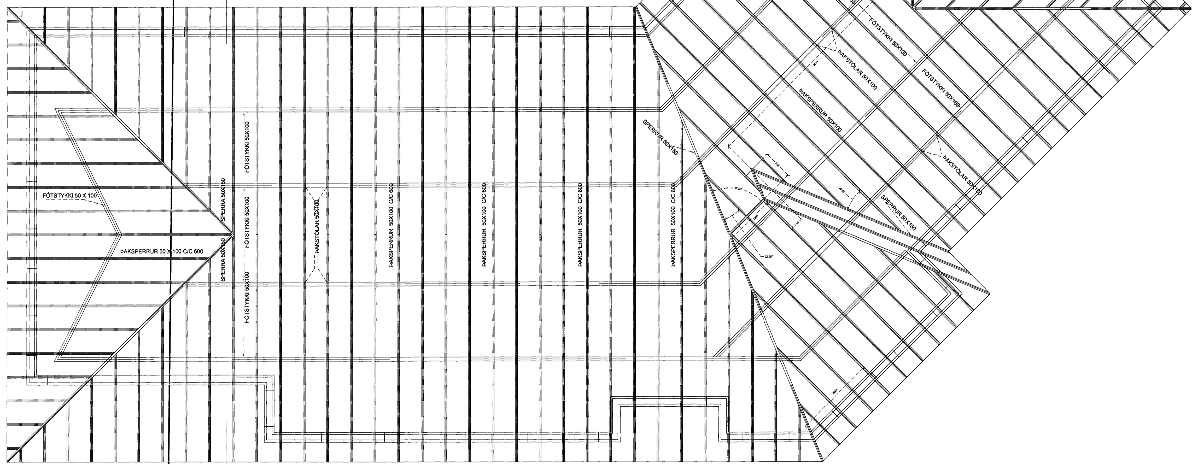
GRUNNMYND ÞAKS MKV 1:50
