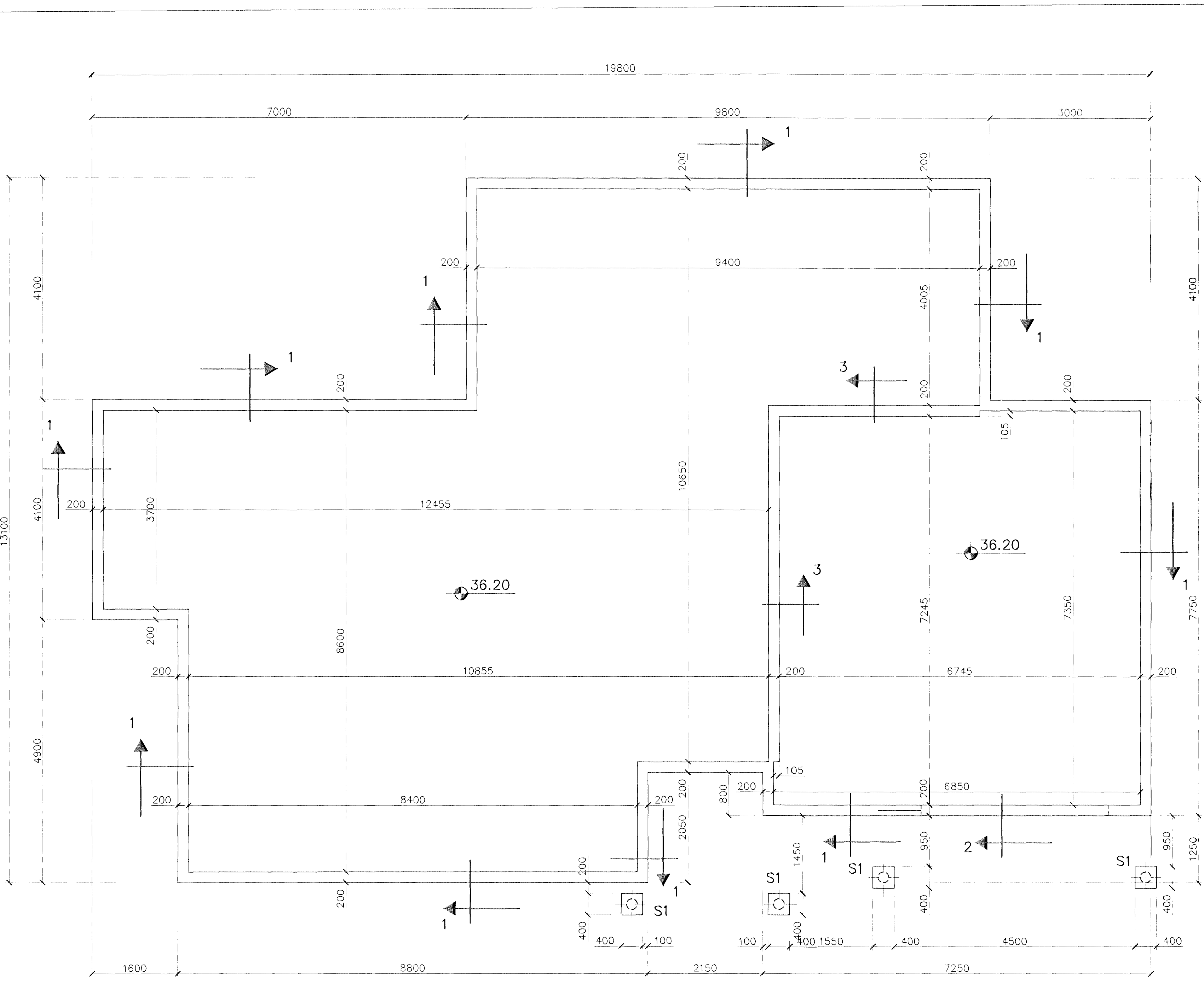
GRUNNMYND 1:50
