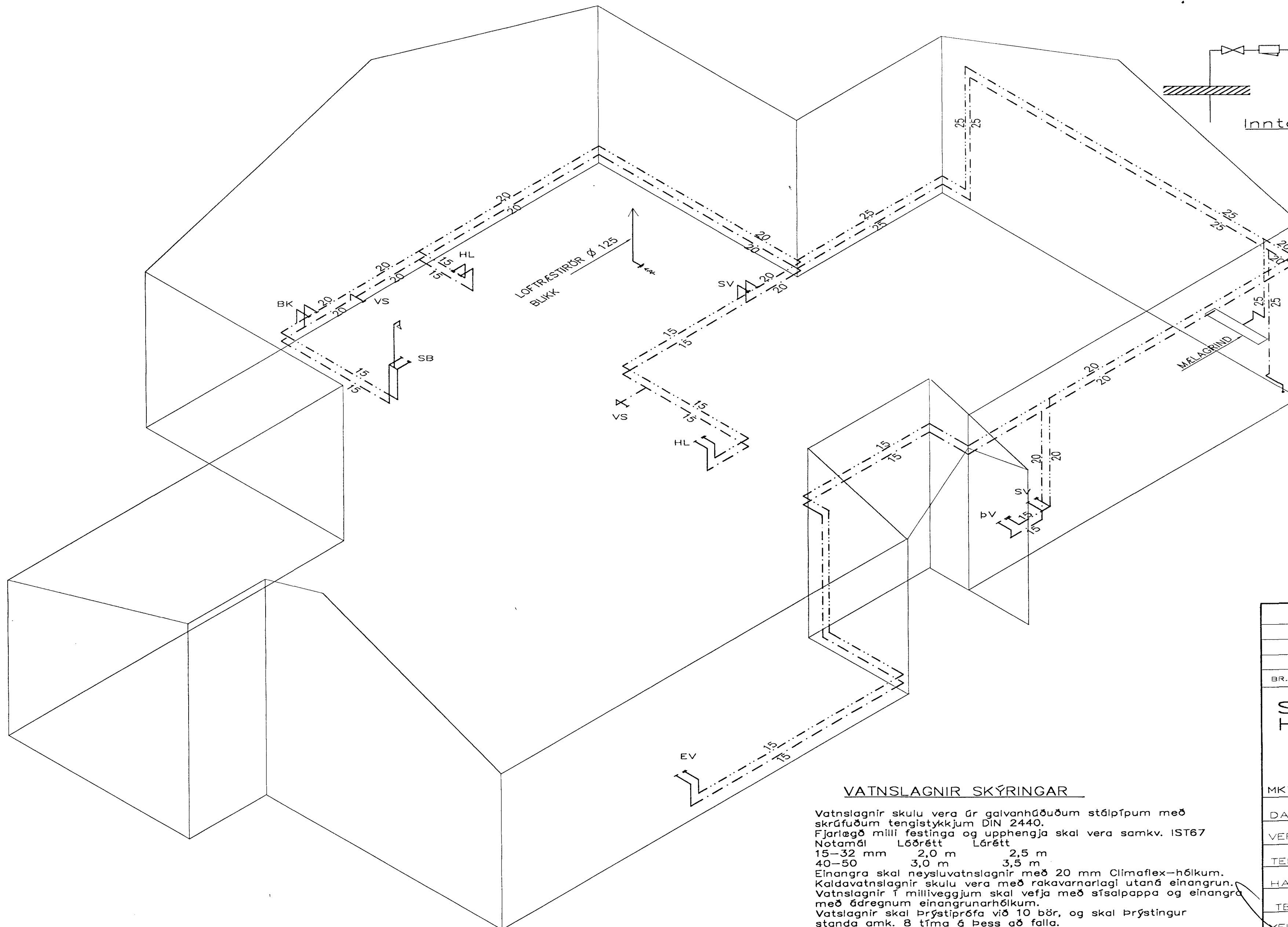
RÚMMYND VATNSLAGNA 1:50
