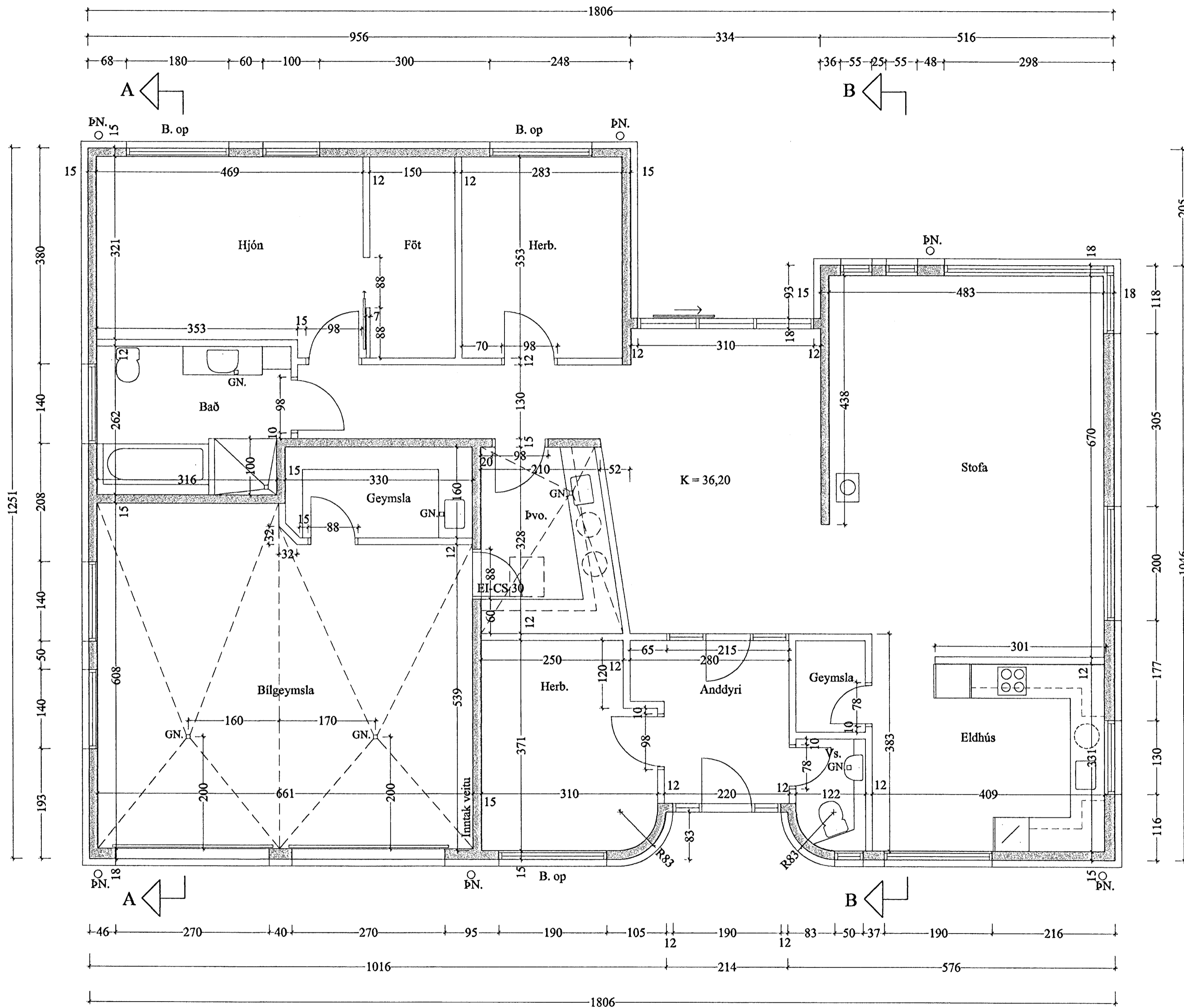
GRUNNMYND M 1:100
