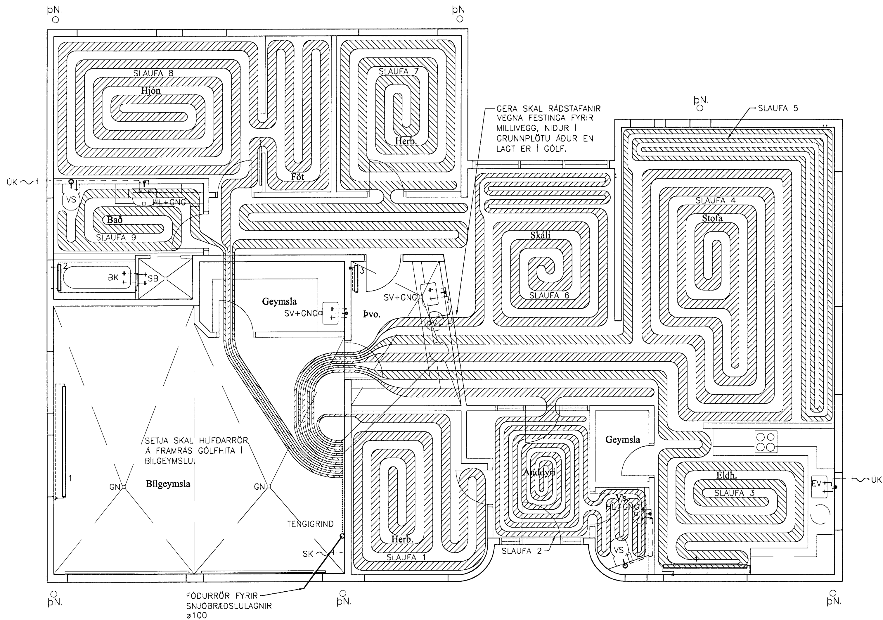
GRUNNMYND 1:50
