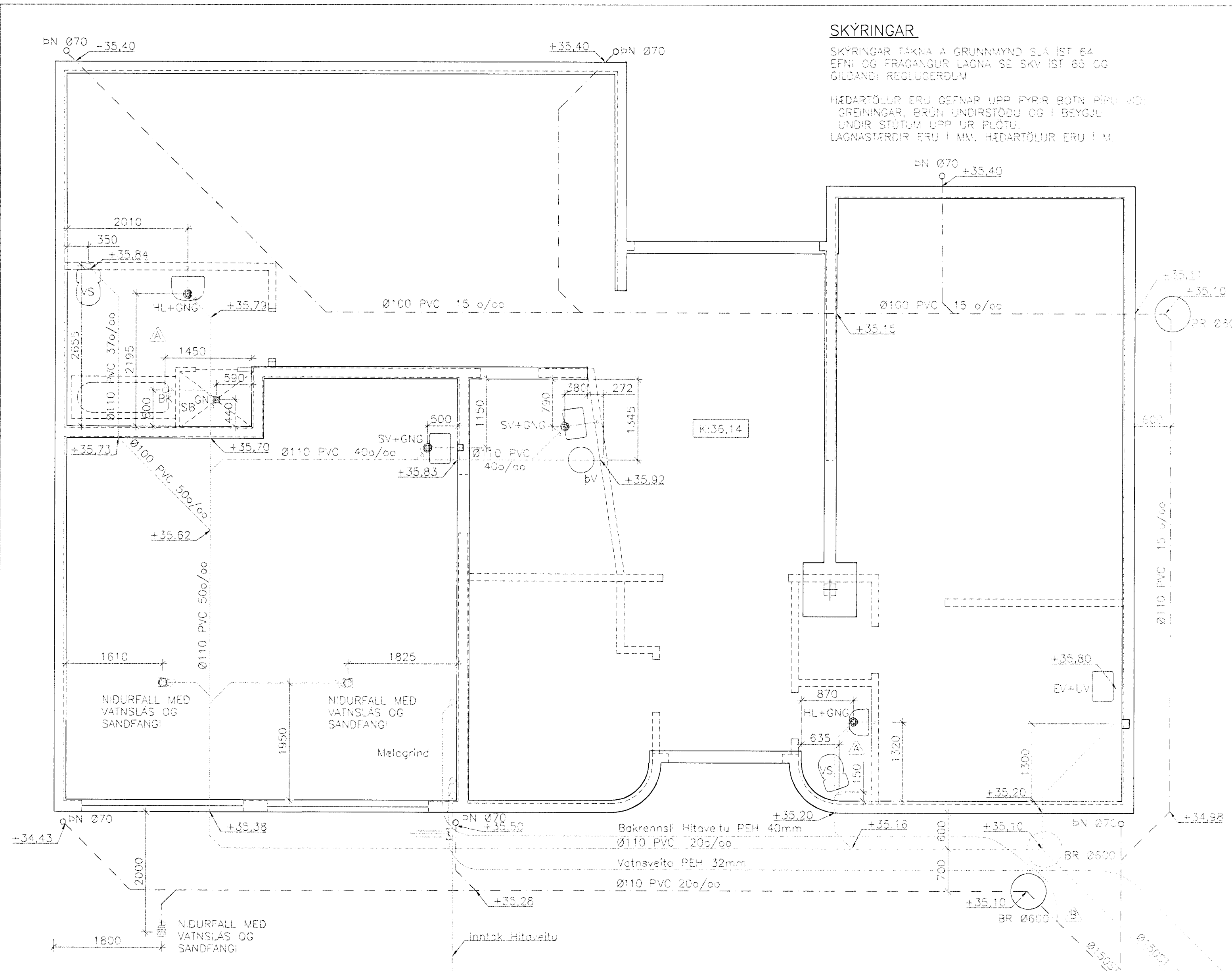
GRUNNMYND Mkv. 1:50
