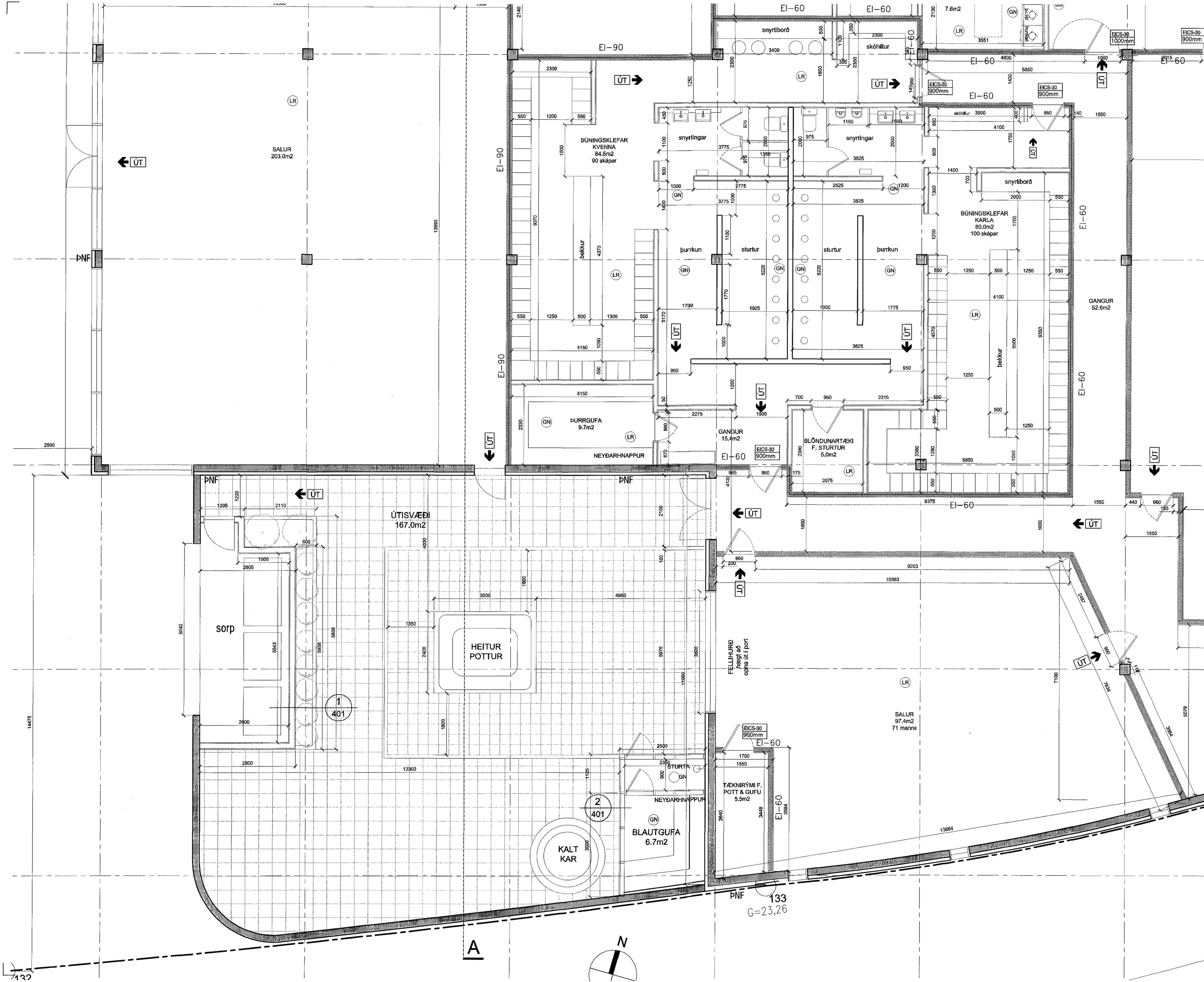
Grunnmynd 1.hæð - Suð-vestur mkv. 1:50
